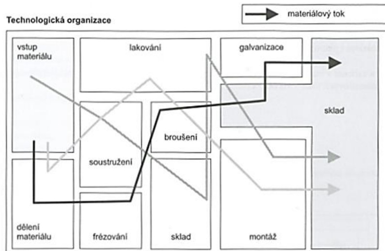
Obrázek č. 5: Technologické uspořádání pracovišť (Zdroj: 3, s. 133)
