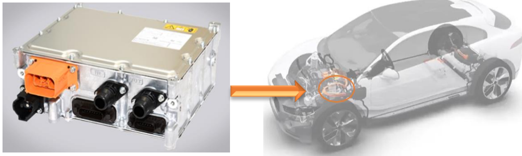
Obrázek č. 17: Palubní nabíjecí jednotka a její umístění v elektromobilu (Zdroj: 27)
