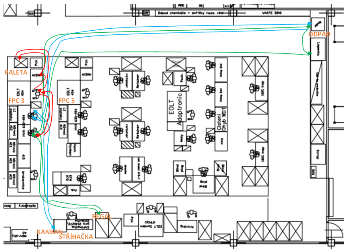
Obrázek č. 39: Nový špagetový diagram operátorů (Zdroj: Vlastní zpracování)
