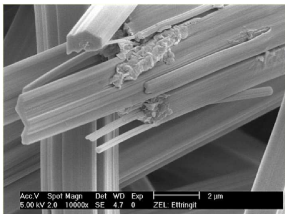
Obrázek 3: Tvar krystalu a mikroskopická struktura ettringitu [7,13]
