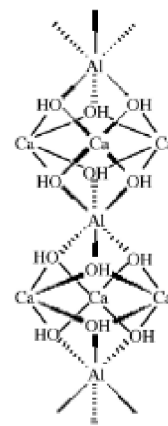
Obrázek 3: Tvar krystalu a mikroskopická struktura ettringitu [7,13]
