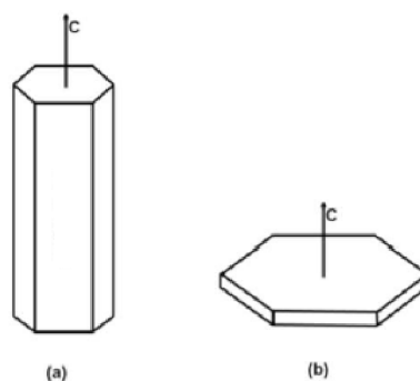
Obránek 1 : Morfologie krystalů a) AFt fáze, b) AFm fáze [36]
