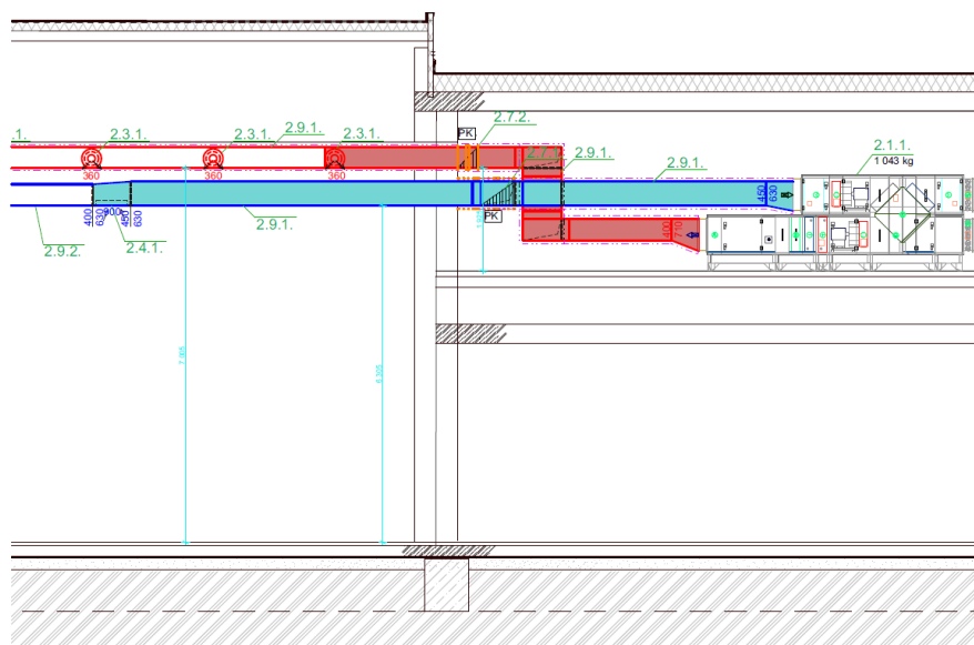
Obr.B. 30 – Vyznačení posuzované trasy k nejbližší přívodní (červená) a odvodní (modrá) vyústce – zař. č. 2
