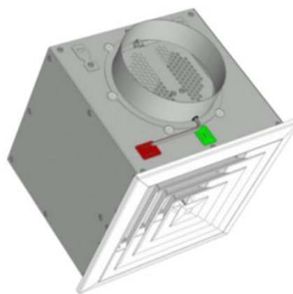
Obr.B. 11 – ALCM s přípojovací skříň – vodorovné připojení 24
