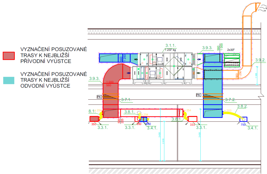
Obr.B. 31 – Vyznačení posuzované trasy k nejbližší přívodní (červená) a odvodní (modrá) vyústce – zař. č. 3
