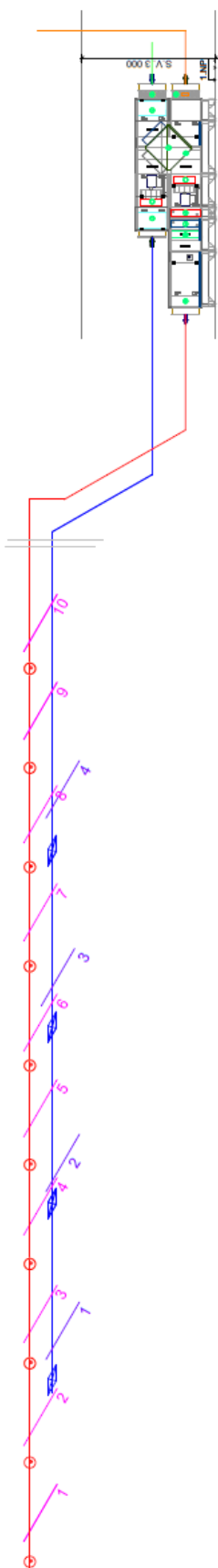
Obr.B. 18 – Axonometrie – Badmintonová hala
