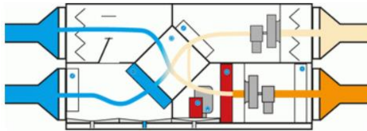
Obr.A. 19 – bazénová jednotka v provozním režimu s cirkulací 18
