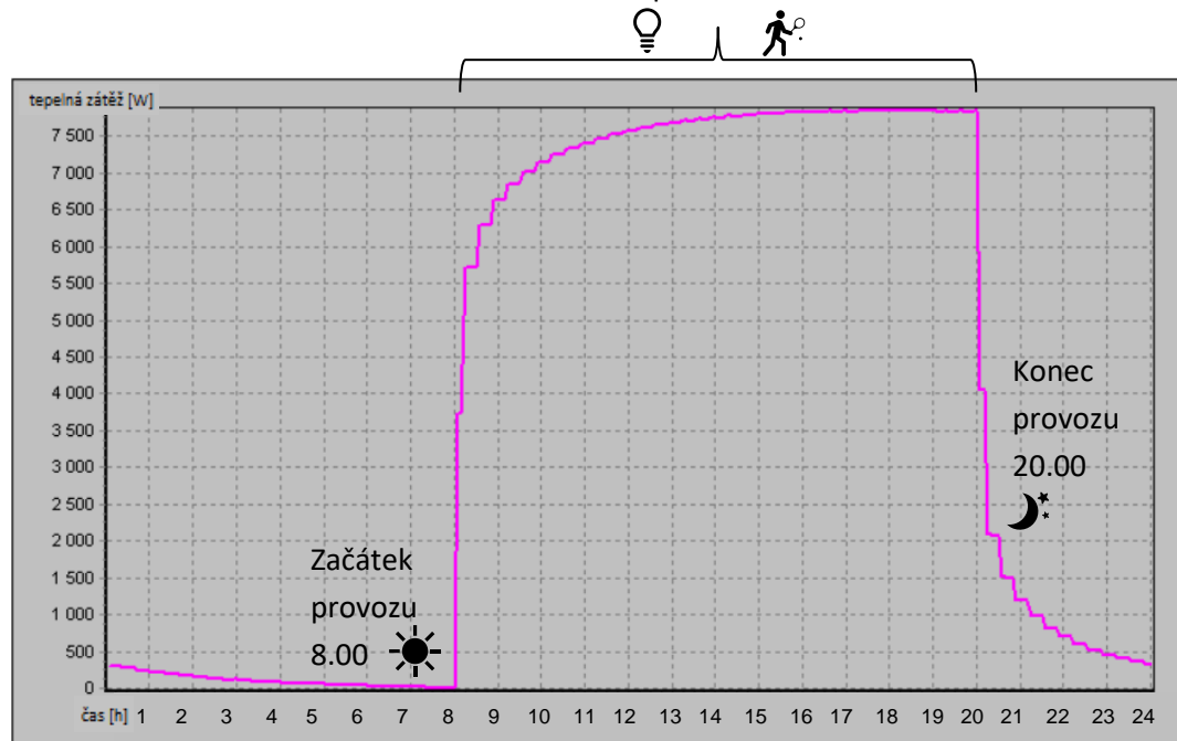
Obr.B. 4 – Graf průběhu tepelné zátěže během dne 39
