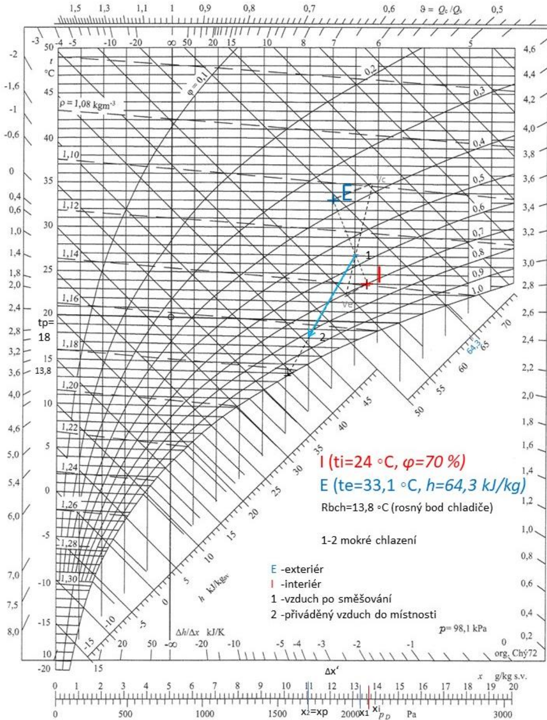
Obr.B. 26 – h - x diagram – LÉTO – Zař. č. 2
