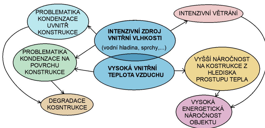
Obr.A. 5 – Schéma okrajových podmínek návrhu bazénových hal z hlediska tepelné techniky 12
