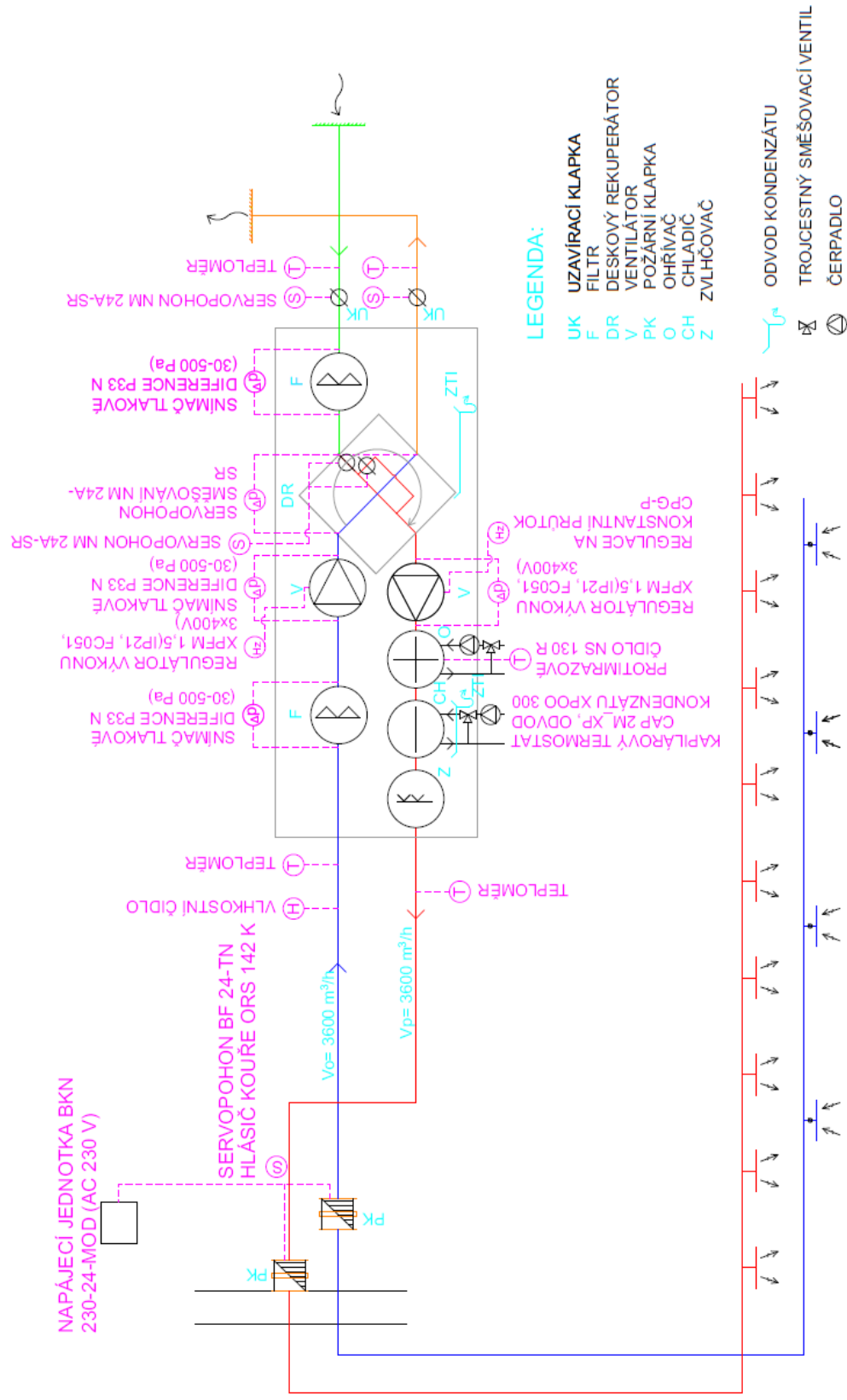
Obr.C. 2 – Funkční schéma zař. č. 2
