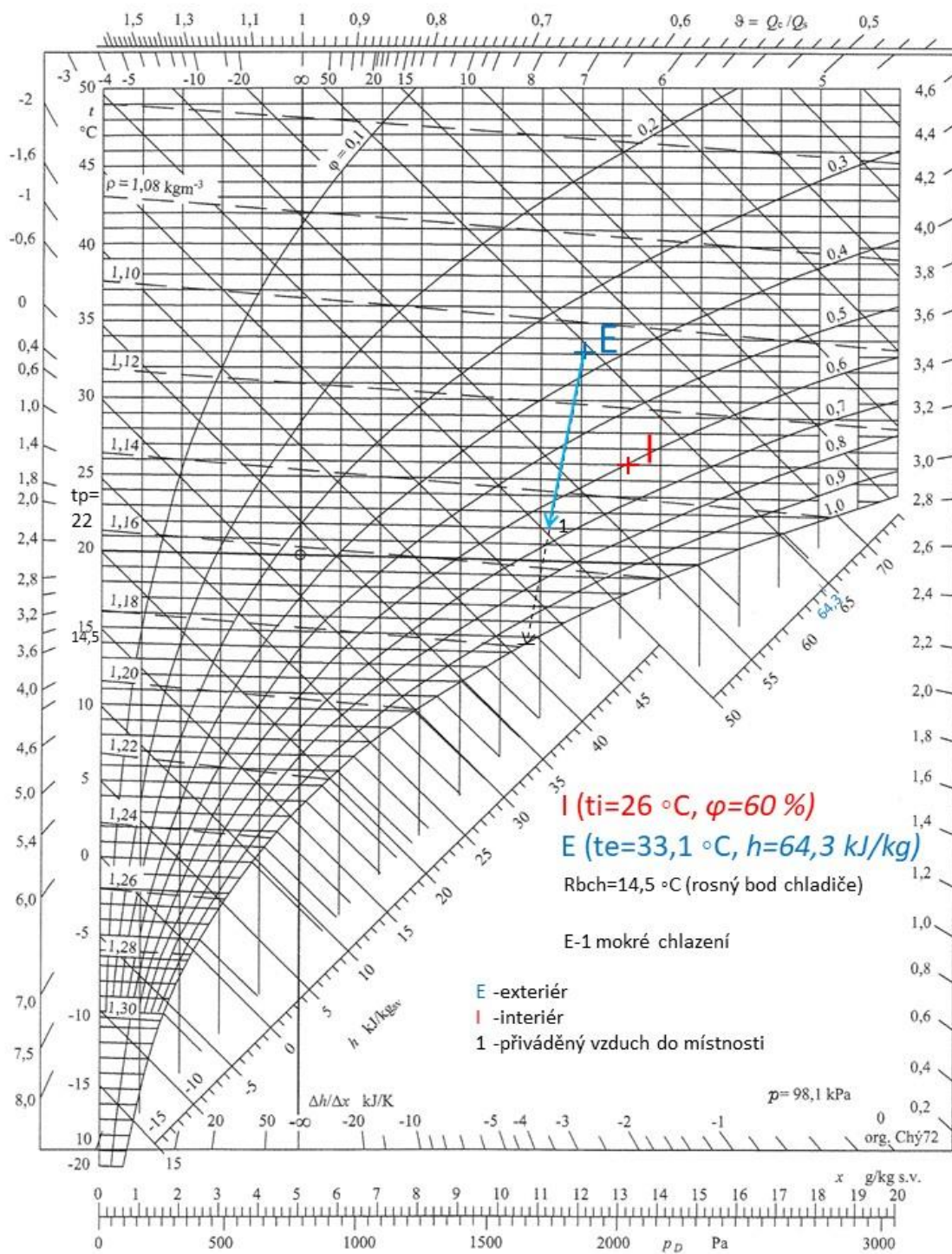
Obr.B. 28 – h-x diagram – ZIMA – Zař. č. 3
