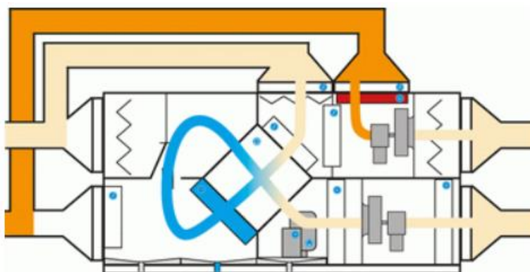
Obr.A. 22 – Upravená bazénová jednotka varianta II. 18
