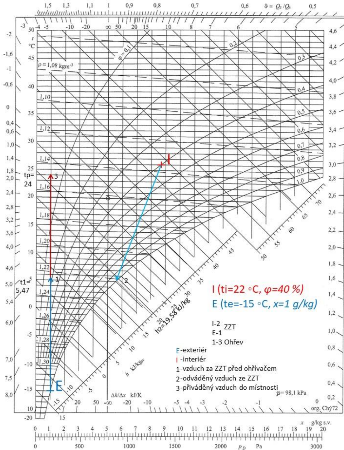
Obr.B. 27 – h-x diagram – ZIMA – Zař. č. 3
