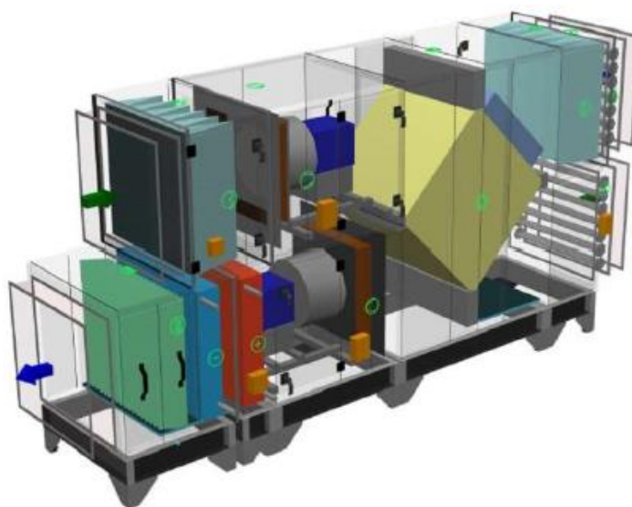
Obr.B. 22 – Axonometrický pohled na zařízení č. 3
