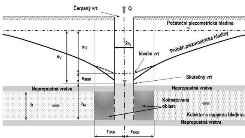
Obrázek 5- Dodatečné odpory na reálném vrtu (KAHUDA et al., 2021)
