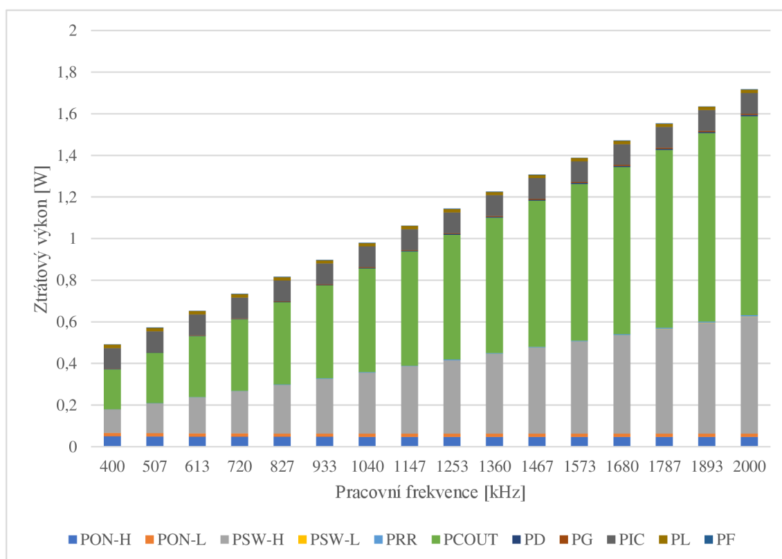
Graf 8: Závislost velikosti ztrát na pracovní frekvenci
