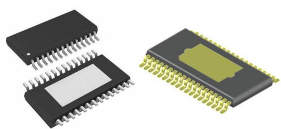
Obrázek 5. Pouzdra integrovaných obvodů, vlevo bottom side a vpravo top side varianta
