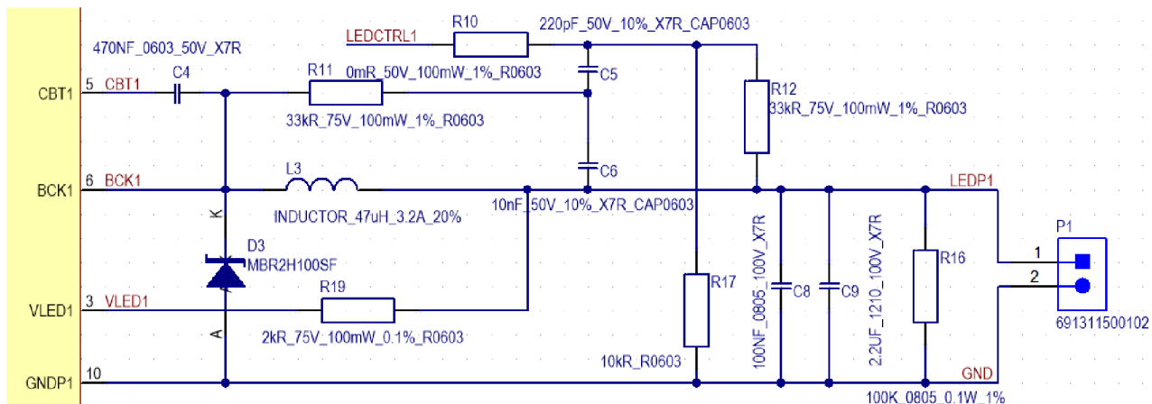
Obrázek 16: Výstupní část snižujícího měniče
