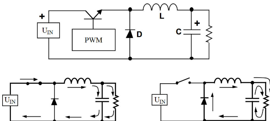
Obrázek 1. Schéma snižujícího měniče [2]
