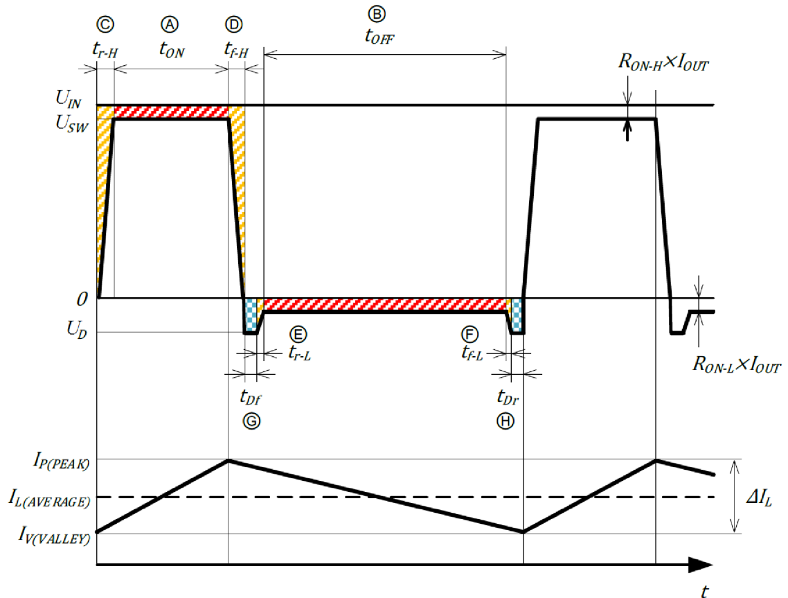
Obrázek 4. Průběhy napětí a proudu na výstupním kontaktu snižujícího měniče. [3]
