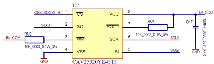
Obrázek 17: Obvod EEPROM
