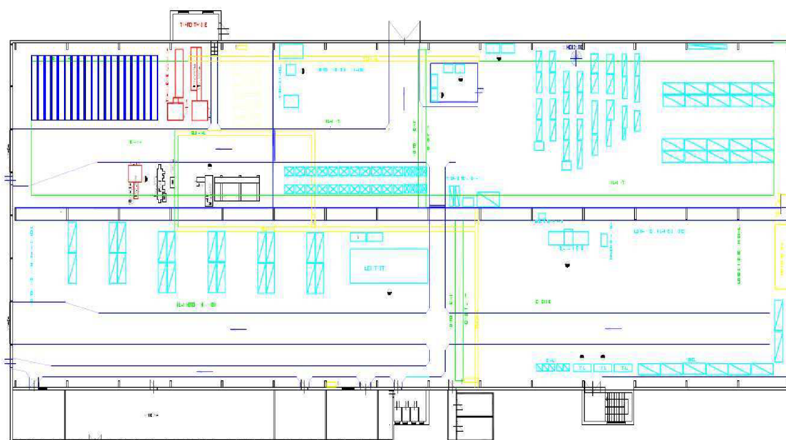
Obr. 2.24 Návrh nové skladovací haly.
