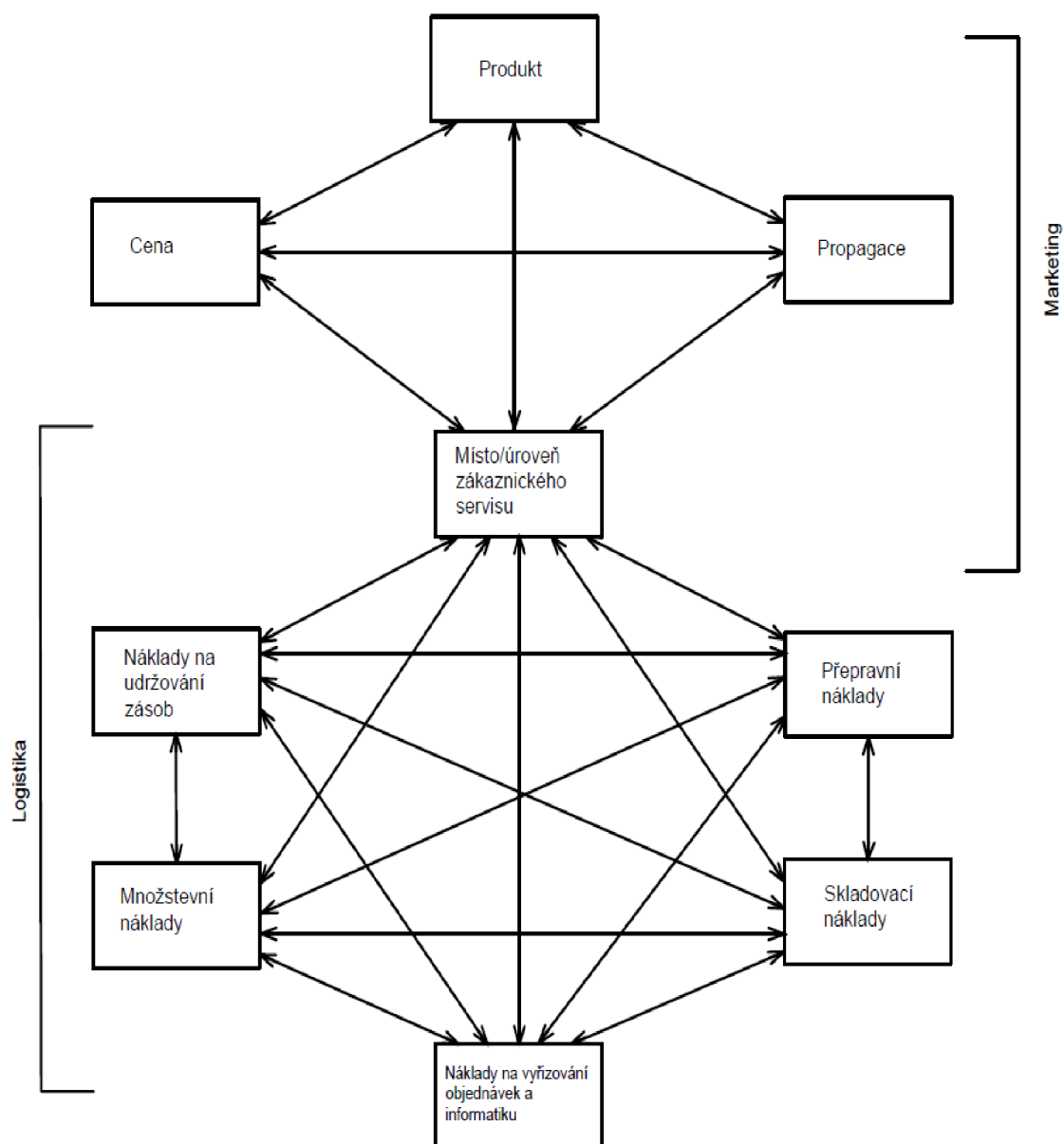
Obr. 1.7 Nákladové vazby. [11]
