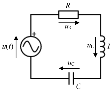
Obr. 2 - Sériovo zapojený RLC obvod.
