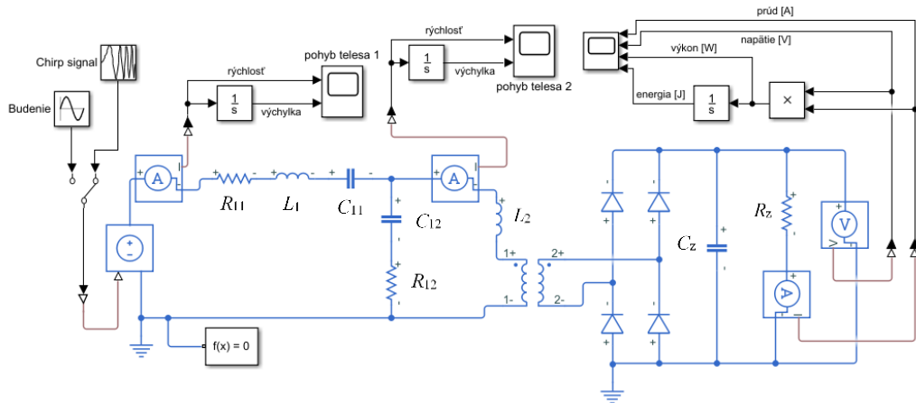
Obr. 28 - Piezoelektrický 2-DOF model generátoru.
