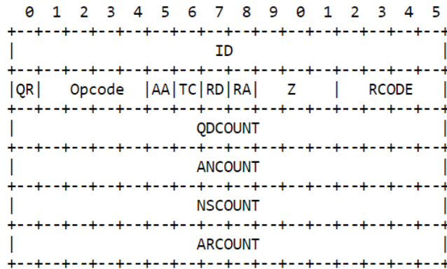
Obrázek 2.4: Hlavička DNS protokolu [7]
