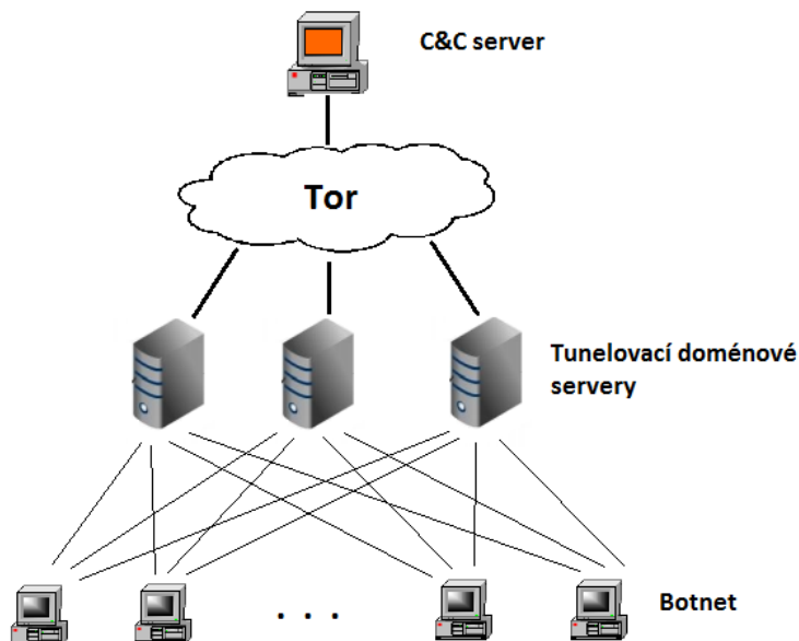
Obrázek 6.2: Architektura botnetu
