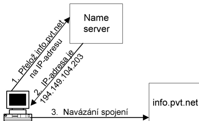
Obrázek 2.1: DNS rezoluce [24]
