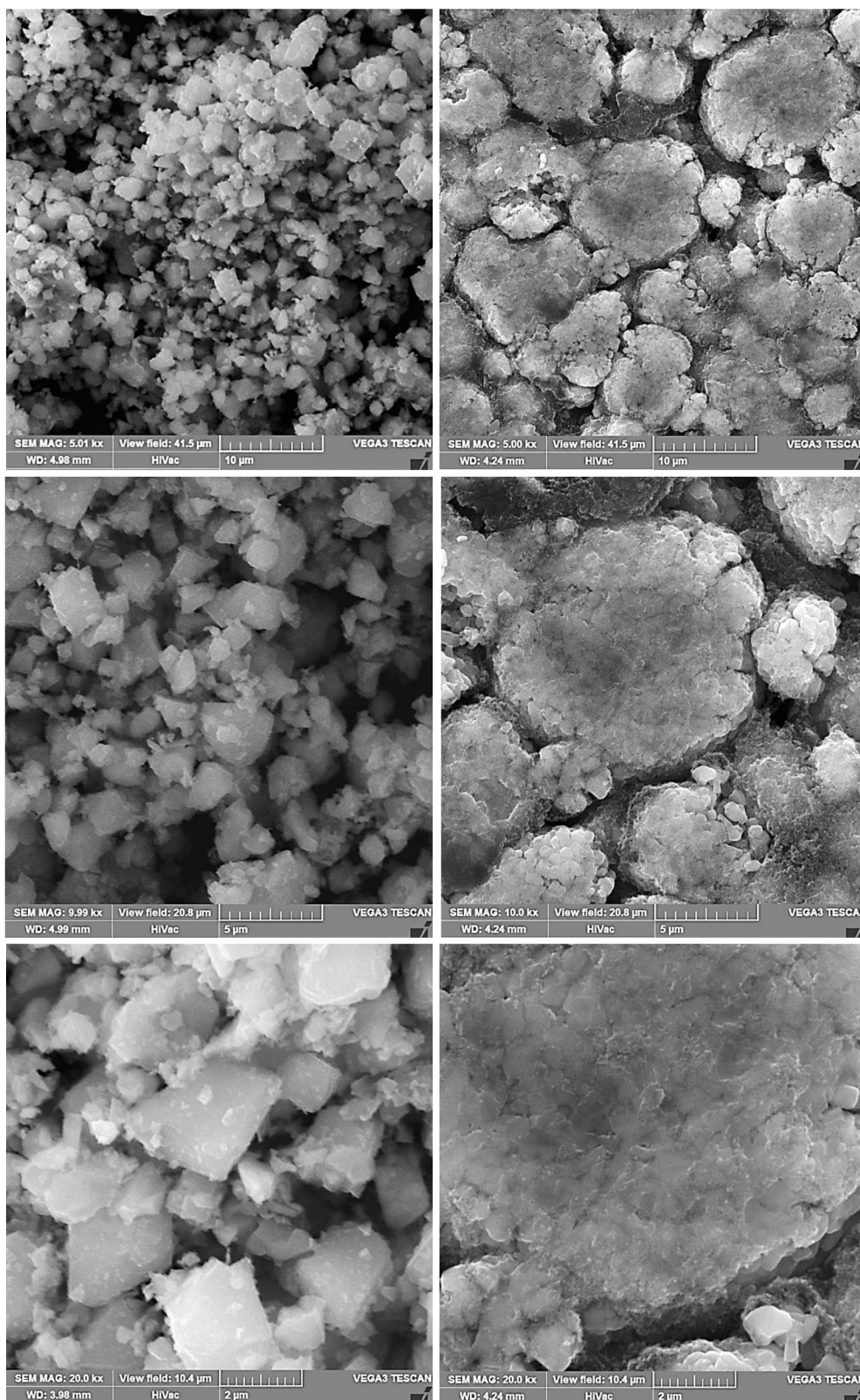
Obrázek 29 Vlevo prášek LNMO a vpravo katodový materiál LCNMO pod elektronovým mikroskopem, zorné pole (FoV) shora 41,5 μm, 20,8 μm, 10,4 μm
