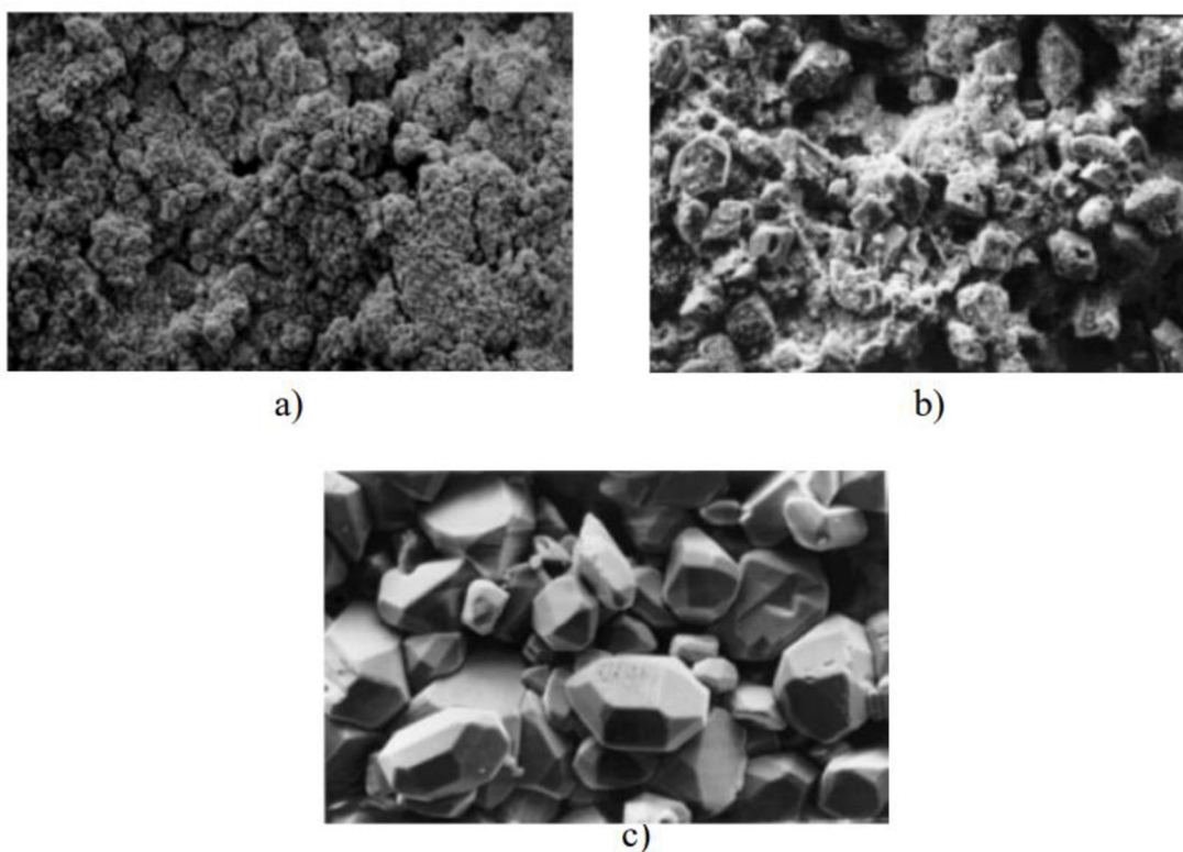
Obrázek 24 Povrch aktivních hmot na elektrodě, zvětšeno 550x: a) bez sulfatace, b) se začínající sulfatací c) s masívní sulfatací [30].
