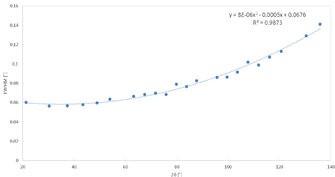
Obrázek 30 Graf se spojnicí trendu pro kompenzaci štěrbinu DS0250
