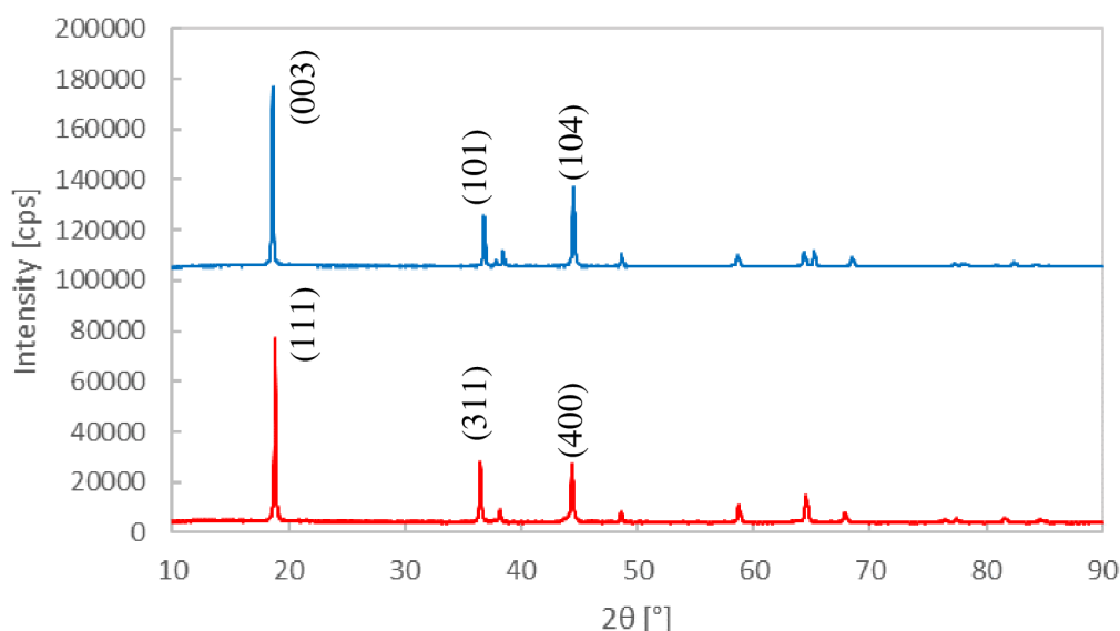
Obrázek 28 Difraktogramy materiálů LCNMO (modře) a LNMO (červeně)
