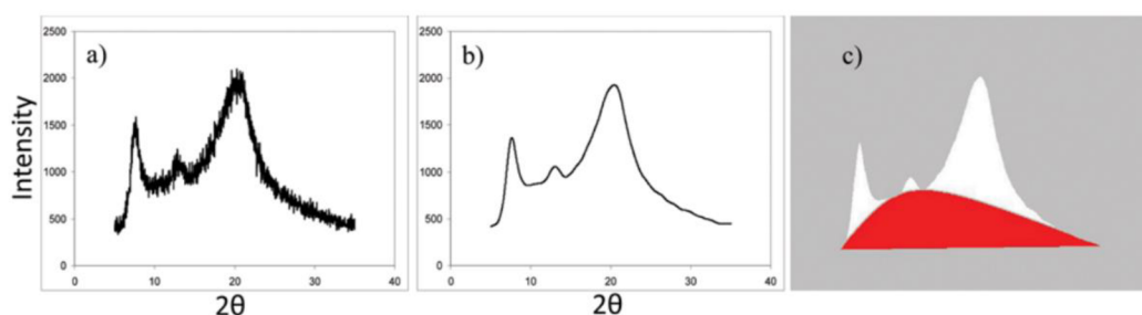
Obrázek 19 a) originální XRD difraktogram, b) vyhlazený pomocí Savitzky-Golayova algoritmu, c) červená část – amorfní složka, bílá část – krystalická složka [24]
