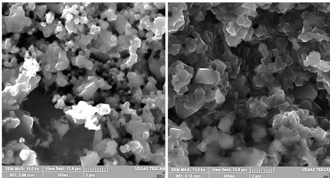
Obrázek 27 Porovnání velikosti krystalů při teplotách kalcinace a) 600 °C, b) 900 °C
