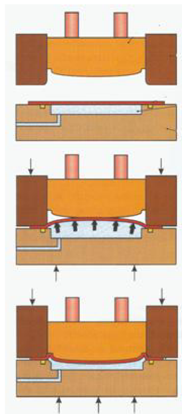
Obr. 13 Fáze hydromechanického tažení [18]
