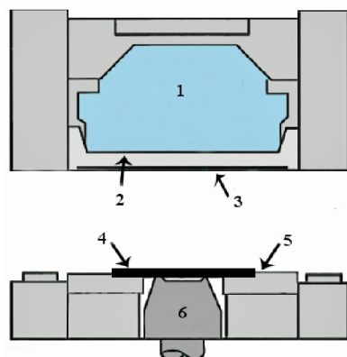
a) Založení polotovaru do nástroje
