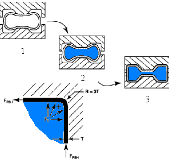
Obr. 30 Fáze postup. hydroformingu [26]
