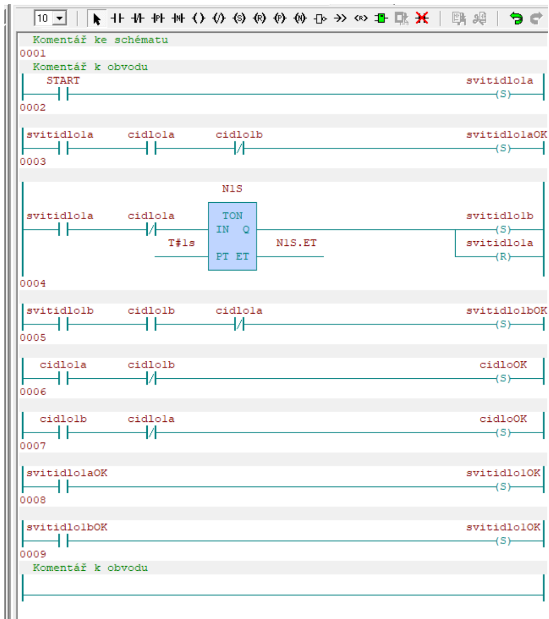
Obr. 4.5: Řídící program
