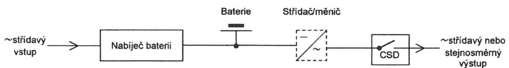
Obr. 1.5: Zapojení s přístrojem pro částečné spínání zátěže [5]
