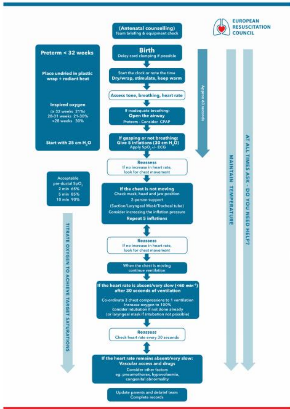
Fig. 5 - NLS algorithm.
