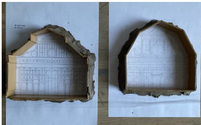
Obrázek 45: Kartonové formy pro odlévání
