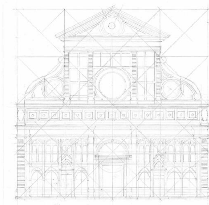
Obrázek 39: Studie průčelí reálné baziliky
