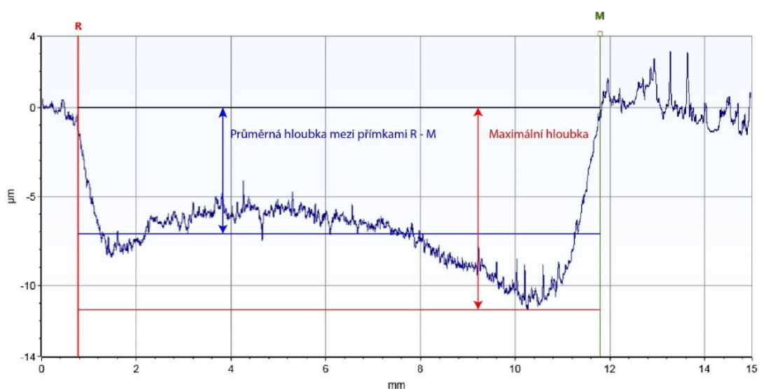
Obr. 3.15 Profil drážky opotřebování
