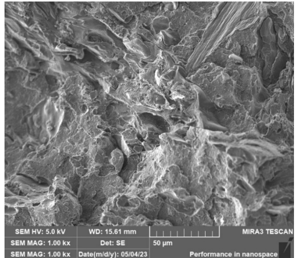
Obr. 4.19 Lomová plocha kompozitu PLLA KM20 po stárnutí
