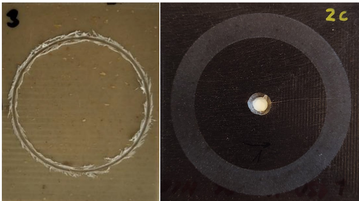
Obr. 4.2 Abrazivní opotřebení vzniklé různými metodami: pin on disk [4] vlevo, taber abraser vpravo
