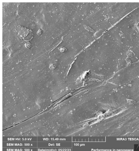
Obr. 4.13 Povrch kompozitu PLLA RH20 po stárnutí
