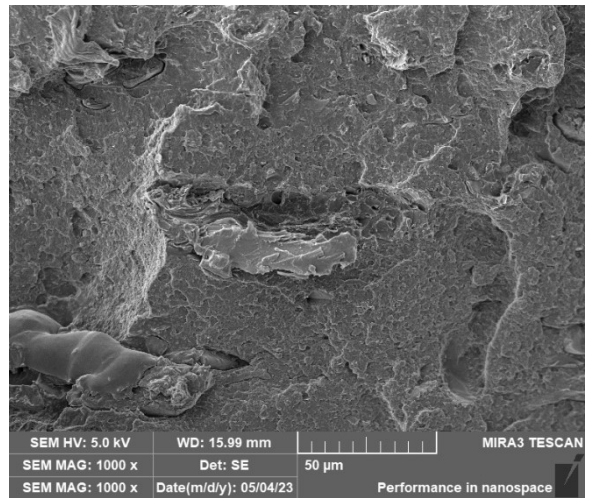
Obr. 4.21 Lomová plocha kompozitu PLLA RH20 po stárnutí
