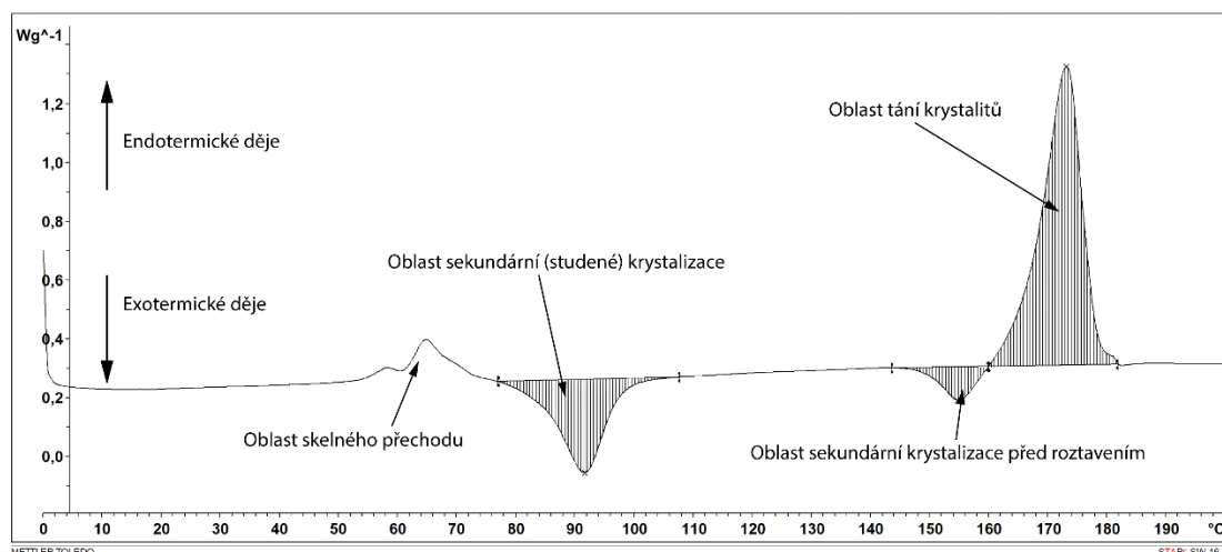
Obr. 3.9 Příklad záznamu DSC křivky pro biokompozit PLLA KM5 ( 10^{\circ}\text{C}\cdot\text{min}^{-1} )
