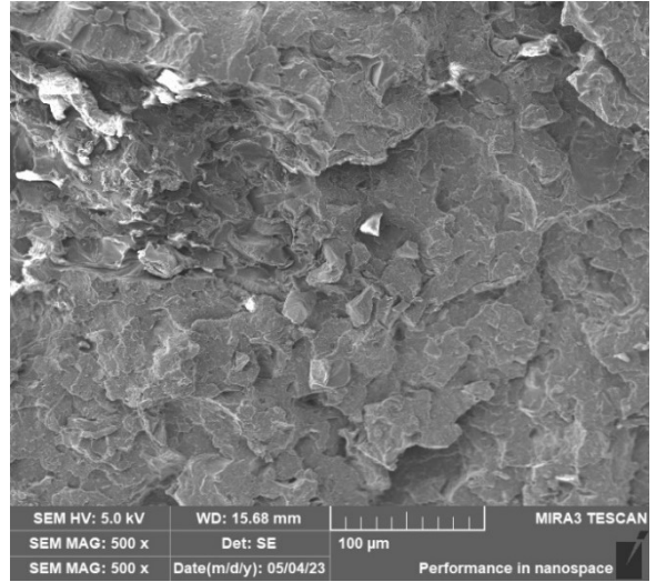
Obr. 4.17 Lomová plocha kompozitu PLLA KN20 po stárnutí
