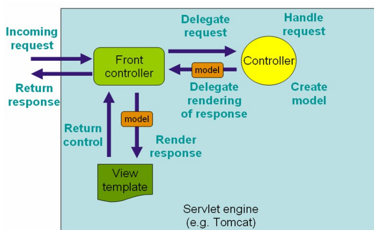
Ilustrace 2.7: Zpracování požadavku ve Spring Web MVC
