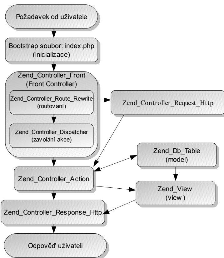
Ilustrace 2.2: Životní cyklus obsluhy požadavku v ZF
