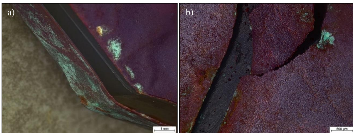
Obr. 43 Povrch struktury z materiálu vstřikovaného PA 12 a) v průběhu klimatického testu (po 5 dnech), b) po ukončení klimatického testu (po 10 dnech)
