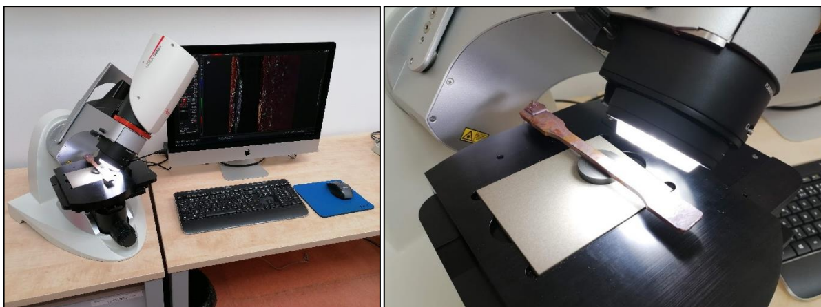
Obr. 23 Digitální optický mikroskop Leica DVM6 (vlevo), detail snímání povrchu kovové vrstvy zkušební tělesa (vpravo)
