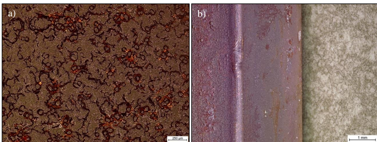
Obr. 44 Povrch struktury polymer – kov před klimatickým testem a) z materiálu PA 12 – MJF, b) z materiálu vstřikovaného PA 12
