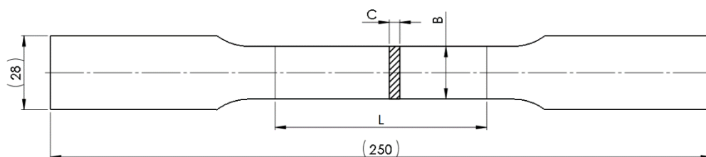
Obr. 33 Náčrt měřených veličin
