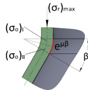
Obr. 21 Schéma ohybových napětí [19]
