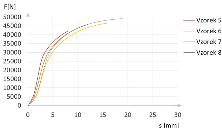
Obr. 37 Závislost tažné síly na dráze příčnicku
