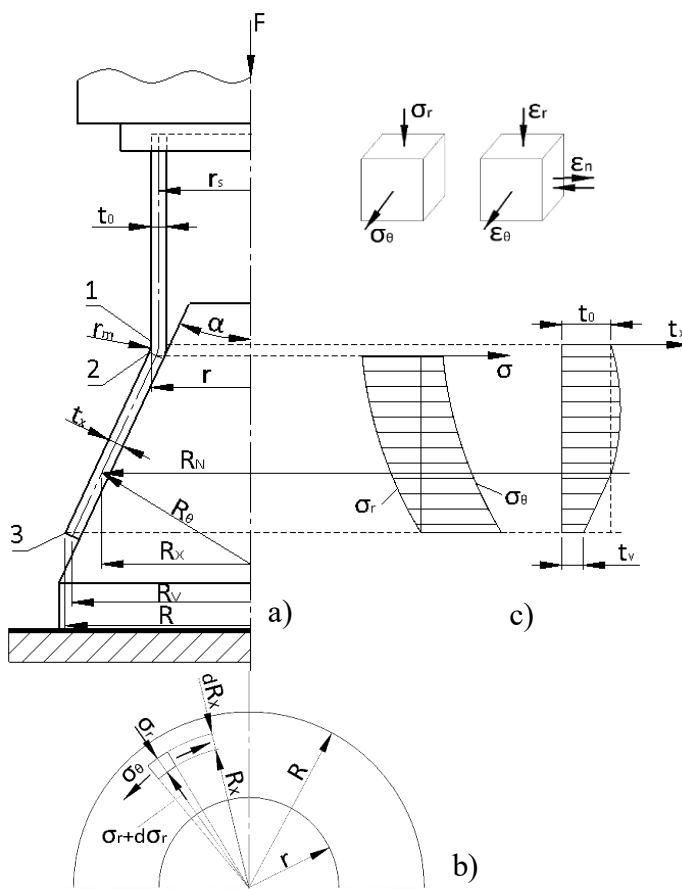
Obr. 18 Schéma principu rozšiřování [17]
