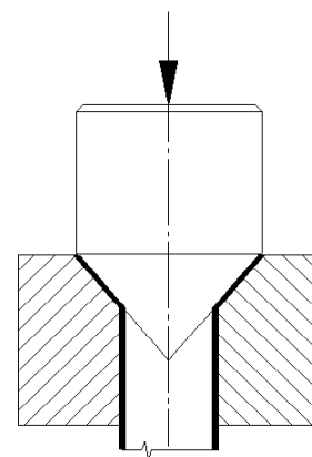
Obr. 12 Schéma s pohyblivým trnem [17]
