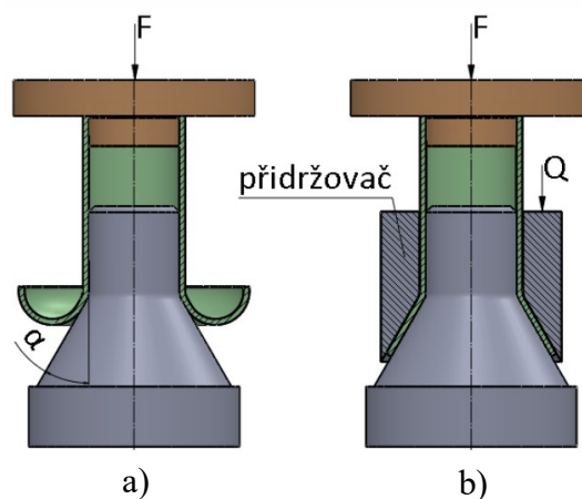
Obr. 25 Vyznačení zakružování [17], [24]
