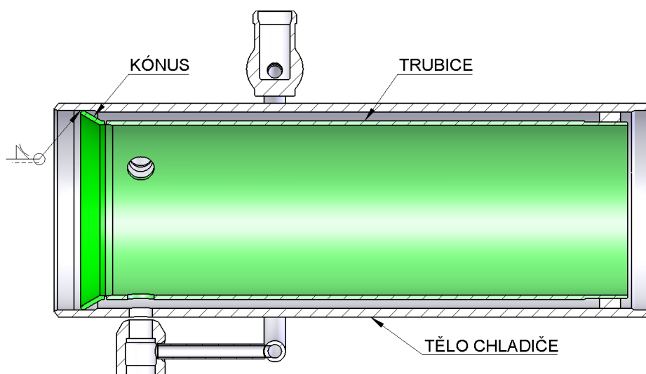
Obr. 3 Svarek chladiče, typ IMI CCI: DAM – 4010/4
