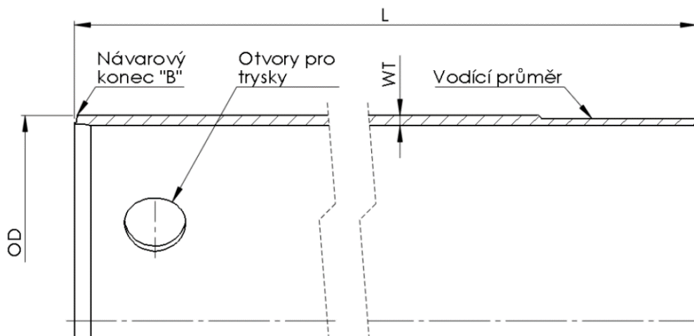
Obr. 5 Trubice
