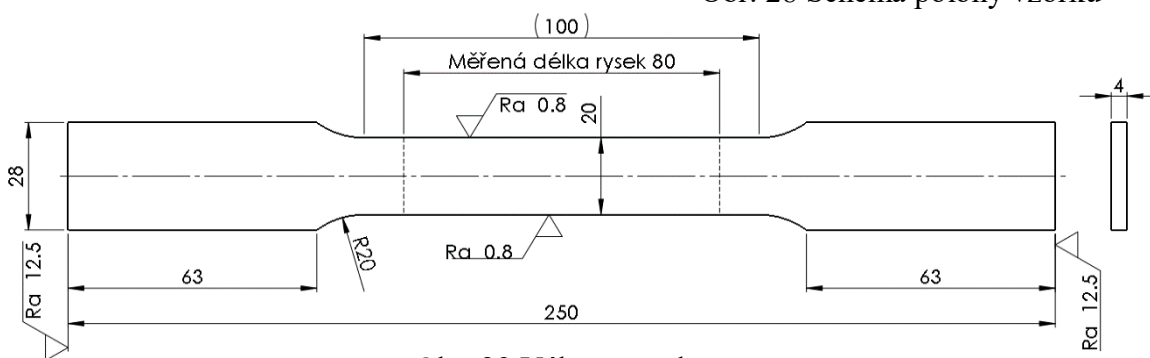
Obr. 29 Výkres vzorku
