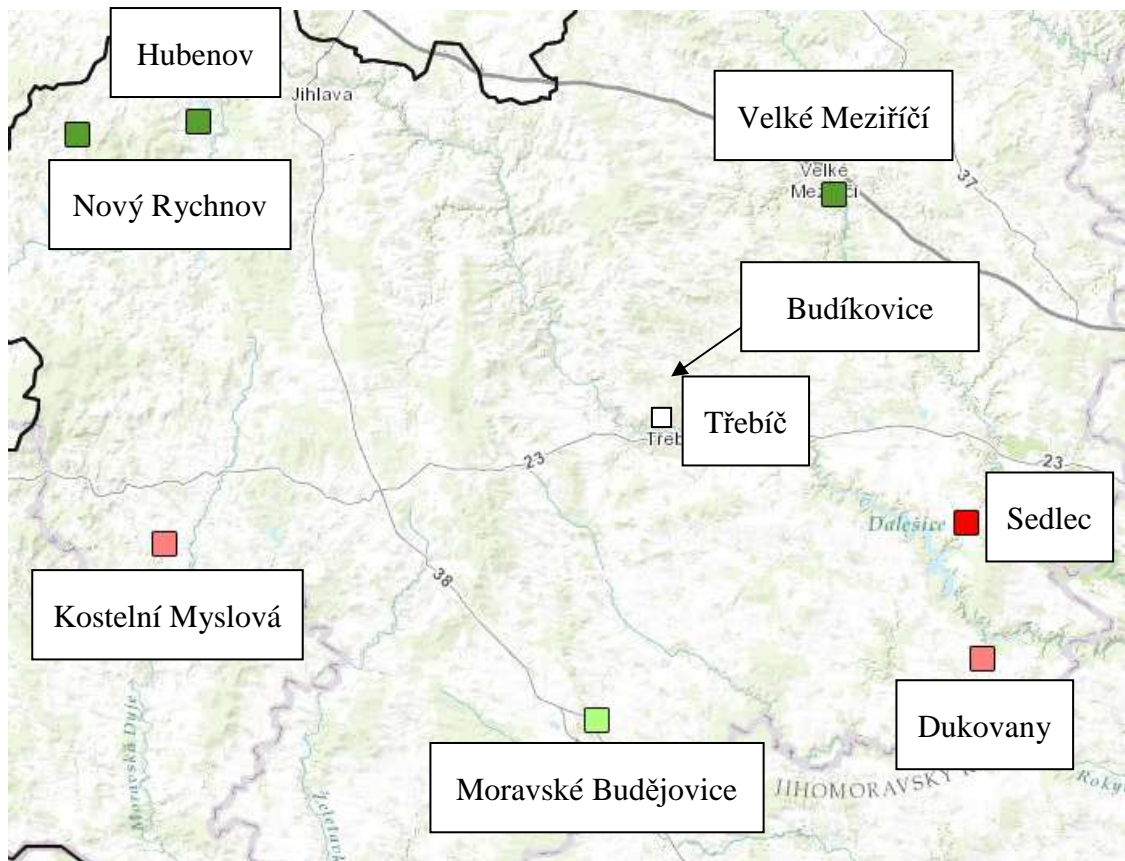
Obr. 3.4 Mapa rozestavení okolních meteorologických stanic
