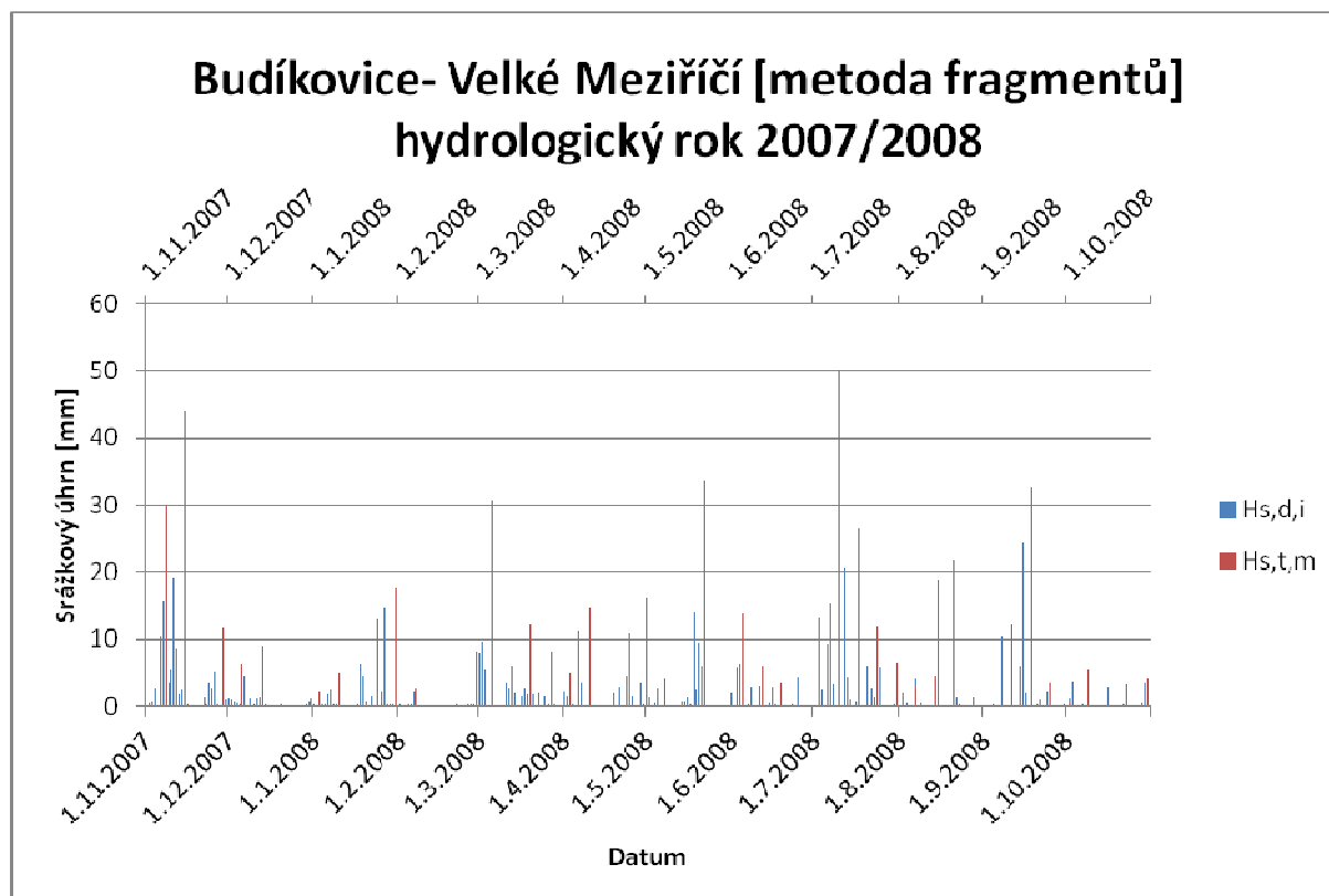
Obř. 3.131 Graf prodloužení řady denních srážkových úhrnů v obci Třebíč/Budíkovice užitím stanice Velké Meziříčí pro hydrologický rok 2007/2008 metodou fragmentů
