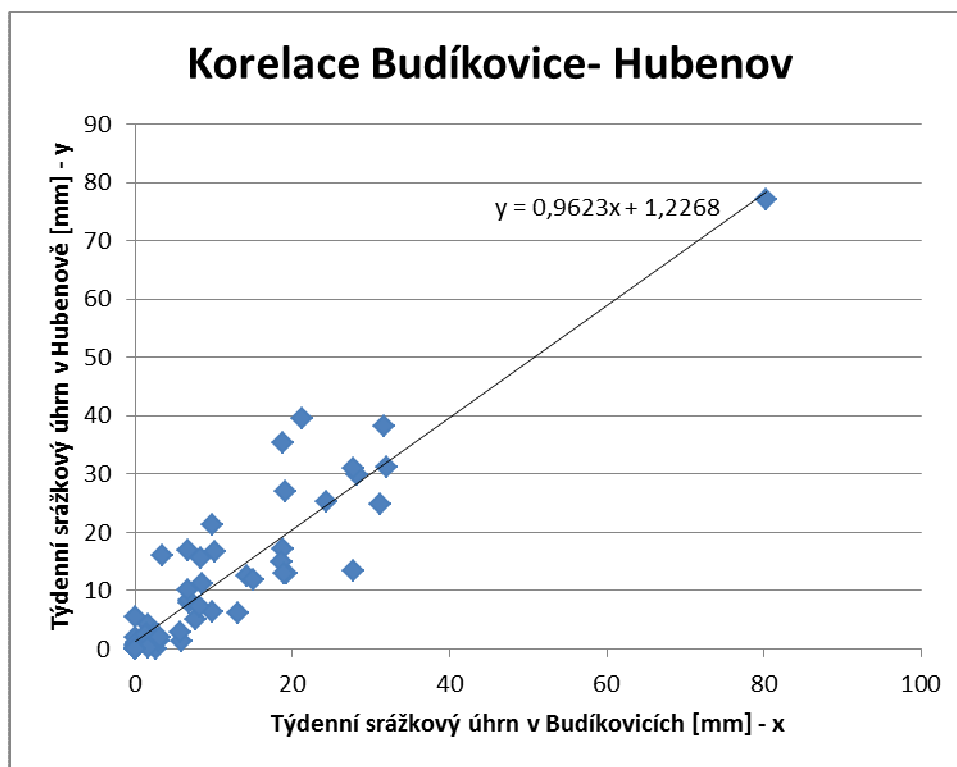
Obr. 3.20 Graf korelace stanic Třebíč/Budíkovice a Hubenov
