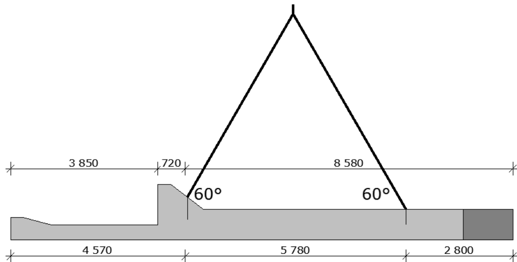
Obr. 5: Rozmístění úchytů pro manipulaci se sloupem ve vertikální poloze
