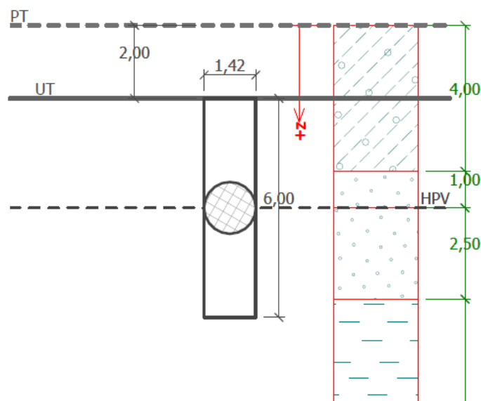
Obr. 1: Profil podloží s vrtanou pilotou
