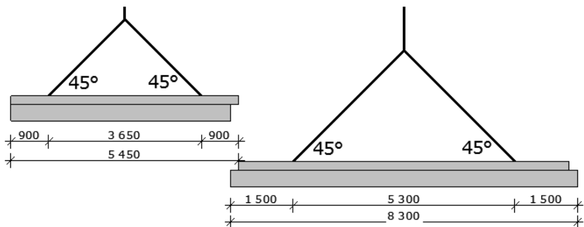
Obr. 7: Rozmístění úchytů pro Gerberův nosník
