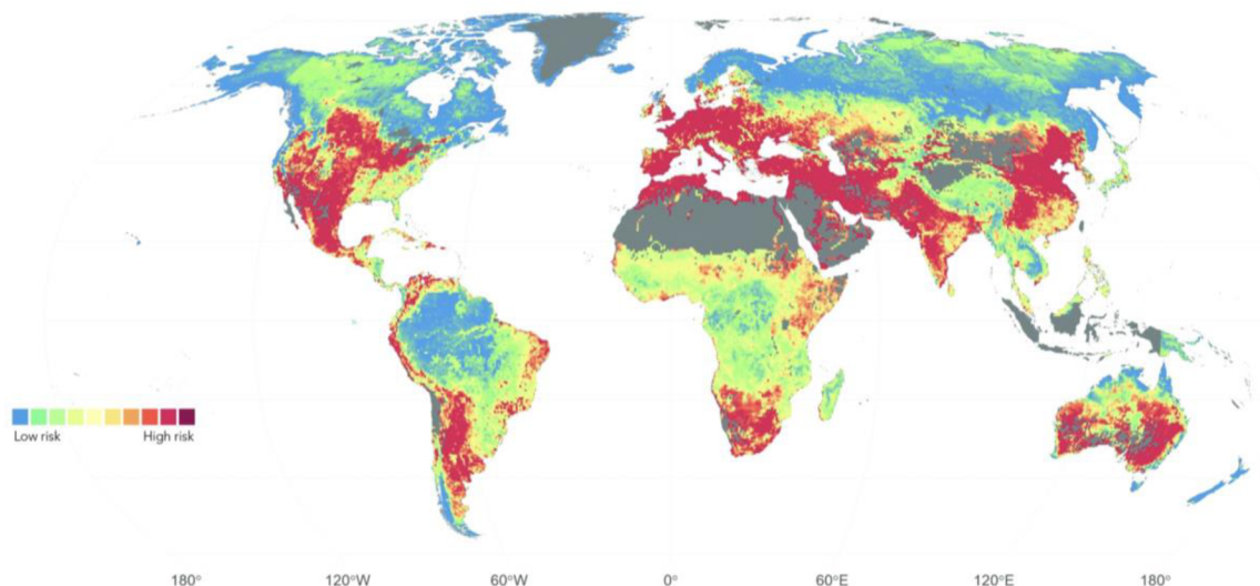
Obr. 4 Rizika pro kvalitu vody v oblasti biologické spotřeby kyslíku, dusíku a elektrické vodivosti
