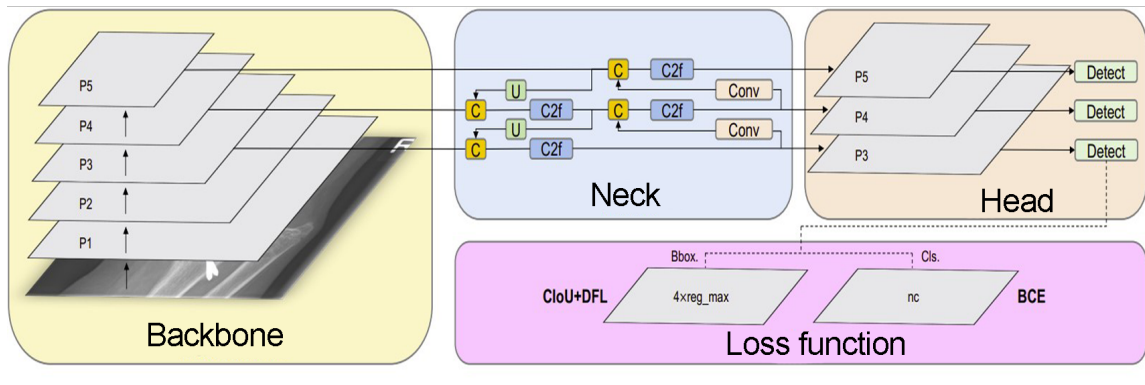
Obr. 2.11: Architektúra modelu YOLOv8, upravené z [30].
