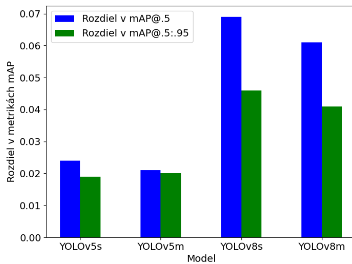
Obr. 4.22: Zlepšenie metrík mAP pri využití hĺbkových dát oproti základným RGB modelom YOLOv5 a YOLOv8.
