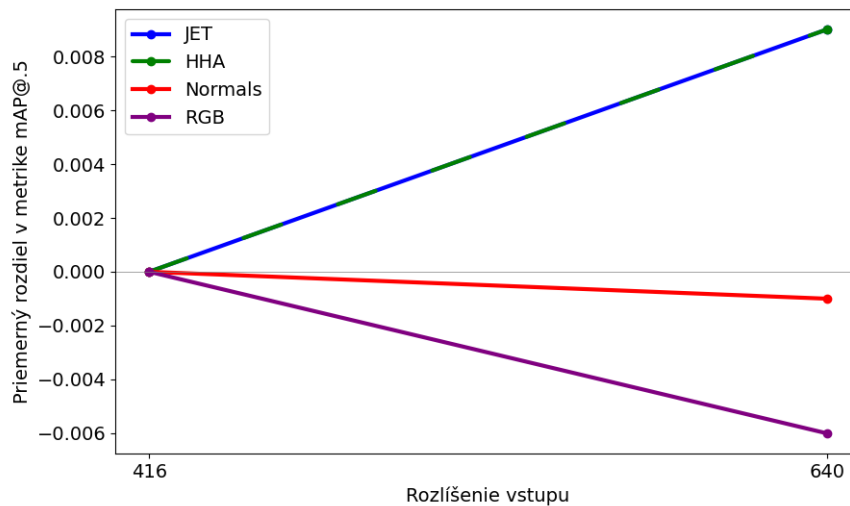
Obr. 4.7: Vplyv zmeny rozlíšenia vstupných obrazov na metriku mAP@.5 väčšieho modelu YOLOv5m využívajúceho metódu skorého zlúčenia.
