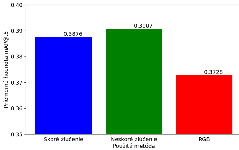
Obr. 4.14: Priemerné hodnoty mAP@.5 rôznych veľkostí modelu a vstupného rozlíšenia podľa metódy zlúčenia.
