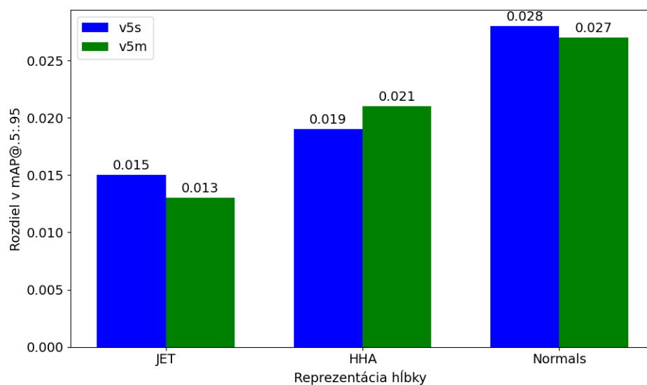
Obr. 4.5: Rozdiel v mAP@.5:.95 medzi modelom využívajúcim metódu skorého zlúčenia a základným RGB modelom pri rozlíšení 640 \times 640 .
