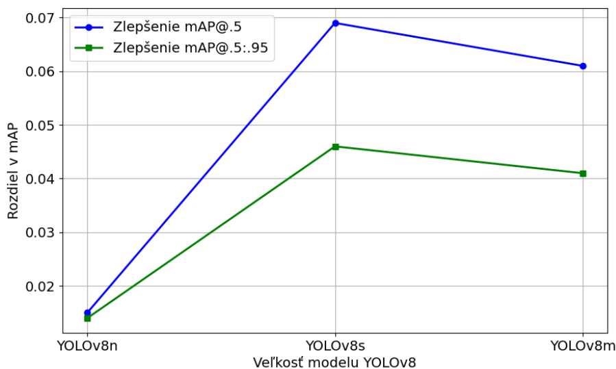
Obr. 4.21: Zlepšenie metrick mAP pri využití hĺbkových dát oproti základným RGB modelom YOLOv8.
