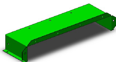
Obr. 31 Pátý ohyb.
