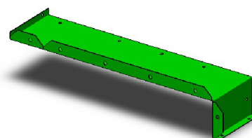
Obr. 30 Čtvrtý ohyb.
