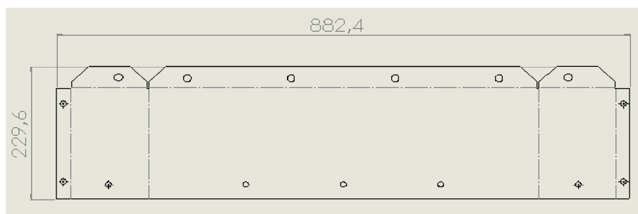
Obr. 23 Rozvinutý tvar.
