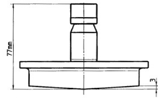
Obr. 7 Razník se šikmým zbroušením. [7]
