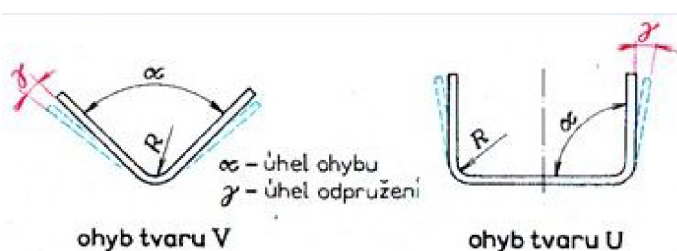
Obr. 15 Odpružení materiálu [4]
