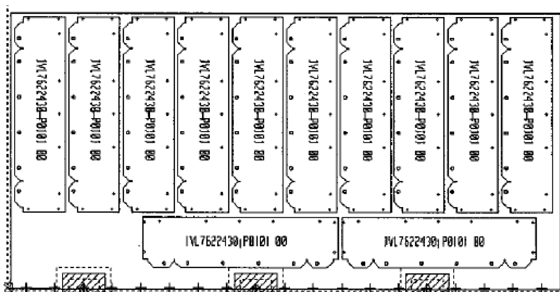
Obr. 25 Nástřihový plán.
