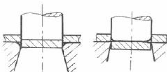
Obr. 6 Stříhání bez vůle (vlevo - kvalitní povrch díry, vpravo - kvalitní povrch výstřížku). [4]
