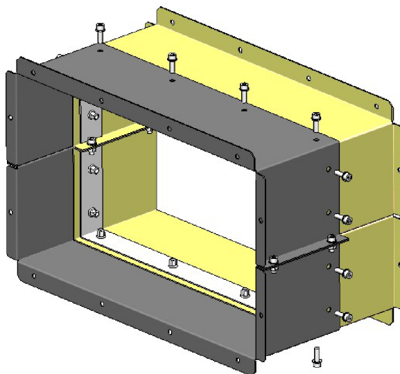
Obr. 38 Kompletní sestava.
