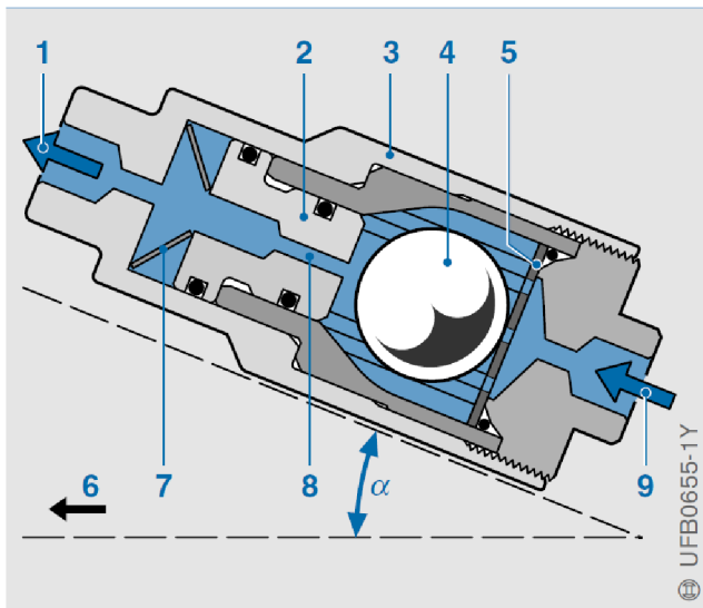
Obrázek 2 Řez tlakovým regulátorem závislým na zrychlení [4]
