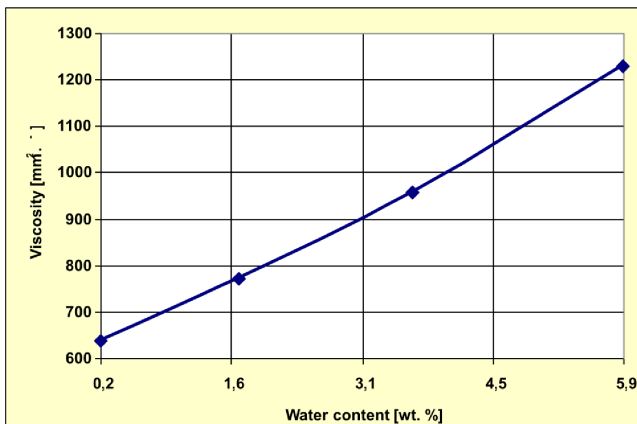
Obrázek 4 Graf závislosti kinematické viskozity na obsahu vody brzdové kapaliny třídy DOT 4 při - 40 °C [28]
