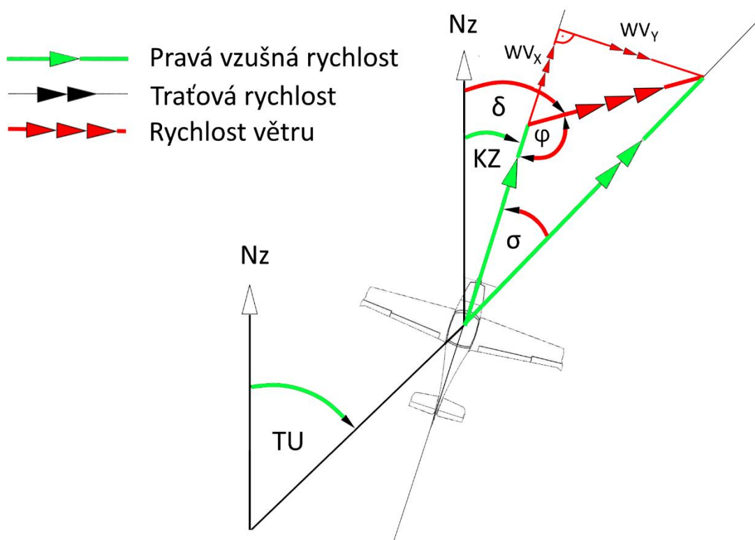
Obr. 22 Znamé a neznámé informace při navigaci pomocí GPS při letu příčně k proudění větru
