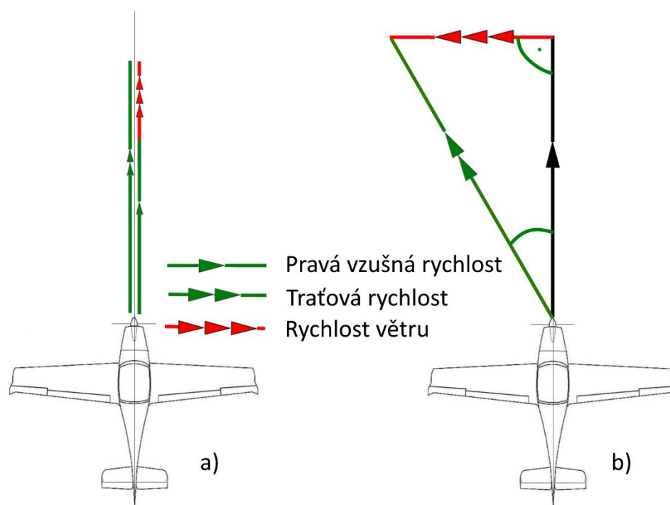
Obr. 21 Známé a neznámé informace při navigaci pomocí GNSS a) rovnoběžně s prouděním větru b) kolmo na proudění větru
