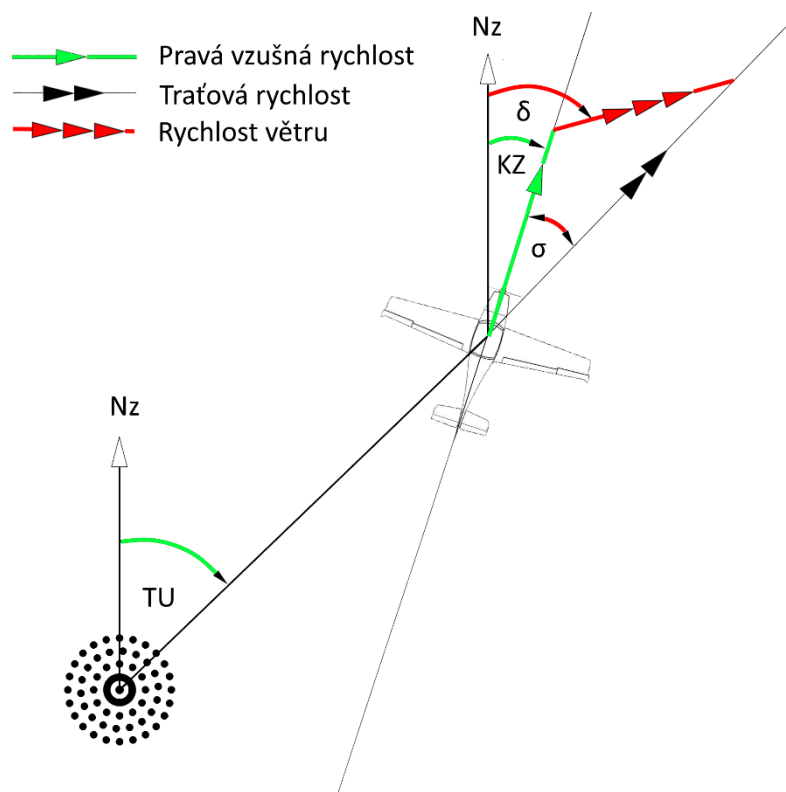
Obr. 17 Známé a neznámé informace při navigaci pomocí NDB
