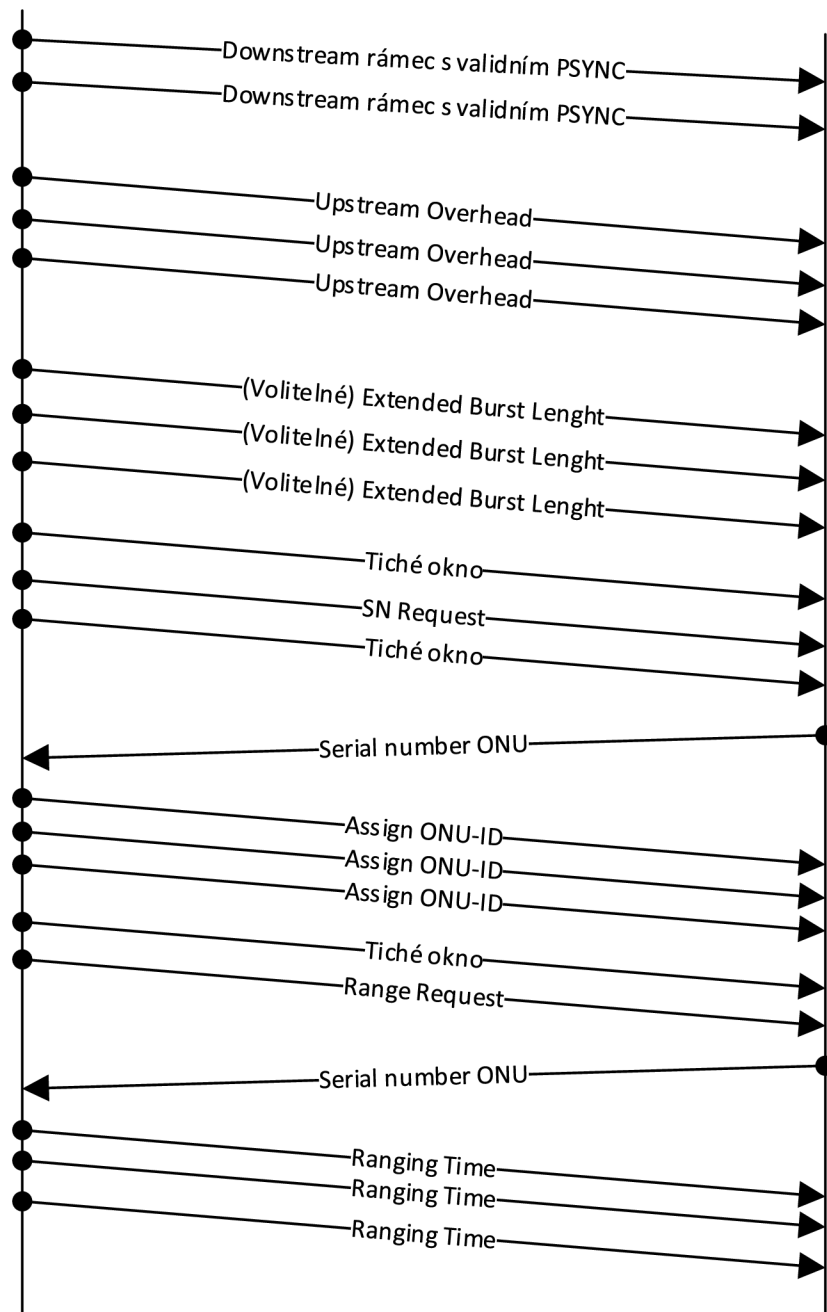
Obr. 6: Aktivační proces [11]
