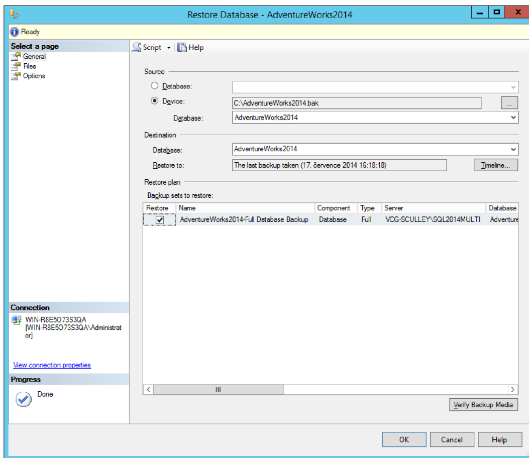
Obr. 11: Obnovení databáze
