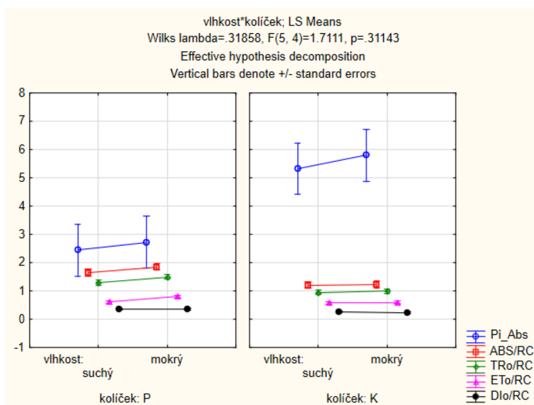
Obr. 21 Analýza rozptylu porovnávající rozdílnost měření na mokré a suché půdě pro hodnoty PI_{ABS} , ABS/RC, TR_0/RC , ET_0/RC , DI_0/RC . Levý graf zobrazuje hodnoty naměřené plochou listovou svorkou (originální); pravý graf kulatou listovou svorkou (vytisknutou). Pravá část grafů vykazuje hodnoty rostlin v mokré půdě; levá na suché. Dle legendy symbolem značíme průměrnou hodnotu a svislicemi 0,95 intervaly spolehlivosti.
