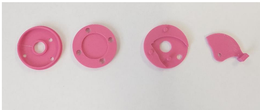
Obr. 14 Přímou vyrobené součástky z 3D tiskárny na konstrukci listové svorky. Po přilepení magnetů a molitanové části, byla získána svorka připravená na jednotlivá měření (Dobšíková, 2023).
