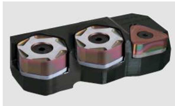
Obr. 1.9 Kazeta s třemi břitovými destičkami [1].
