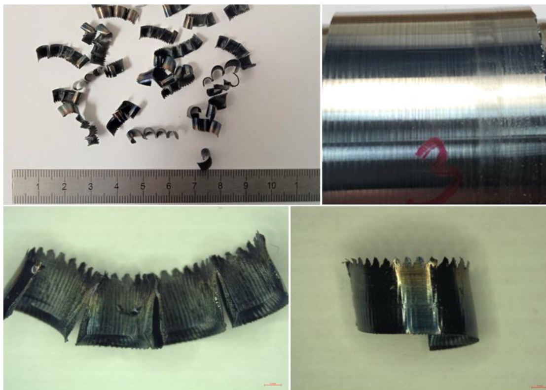
Obr. 3.26 Třísky a obroběný povrch, VBD 3
