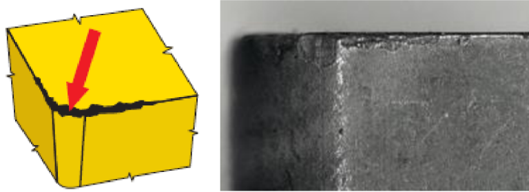
Obr. 2.13 Vylamování částic břitu [1; 2].
