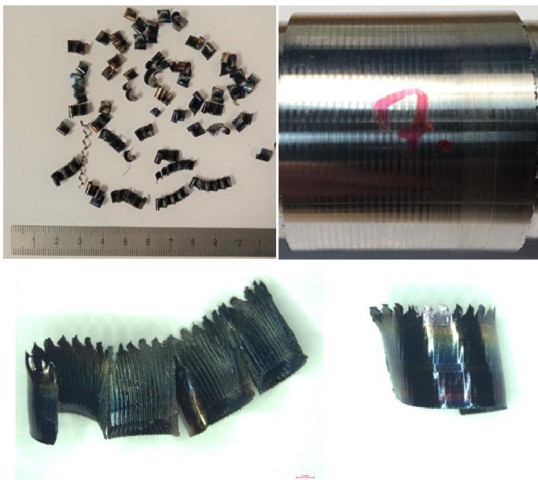
Obr. 3.30 Třísky a obrobený povrch, VBD 7.
