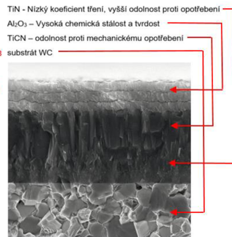
Obr. 2.18 Vícevrstvý povlak [1].
