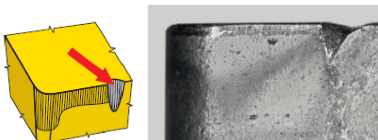
Obr. 2.12 Vrubové opotřebení [1; 2].
