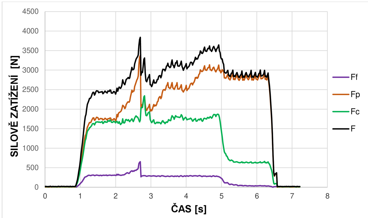
Obr. 3.34 Silové zatížení, VBD 1.
