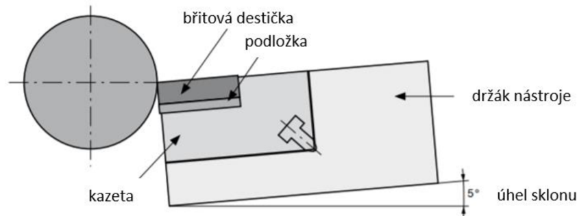
Obr. 1.13 Úhel sklonu břitové destičky [1].
