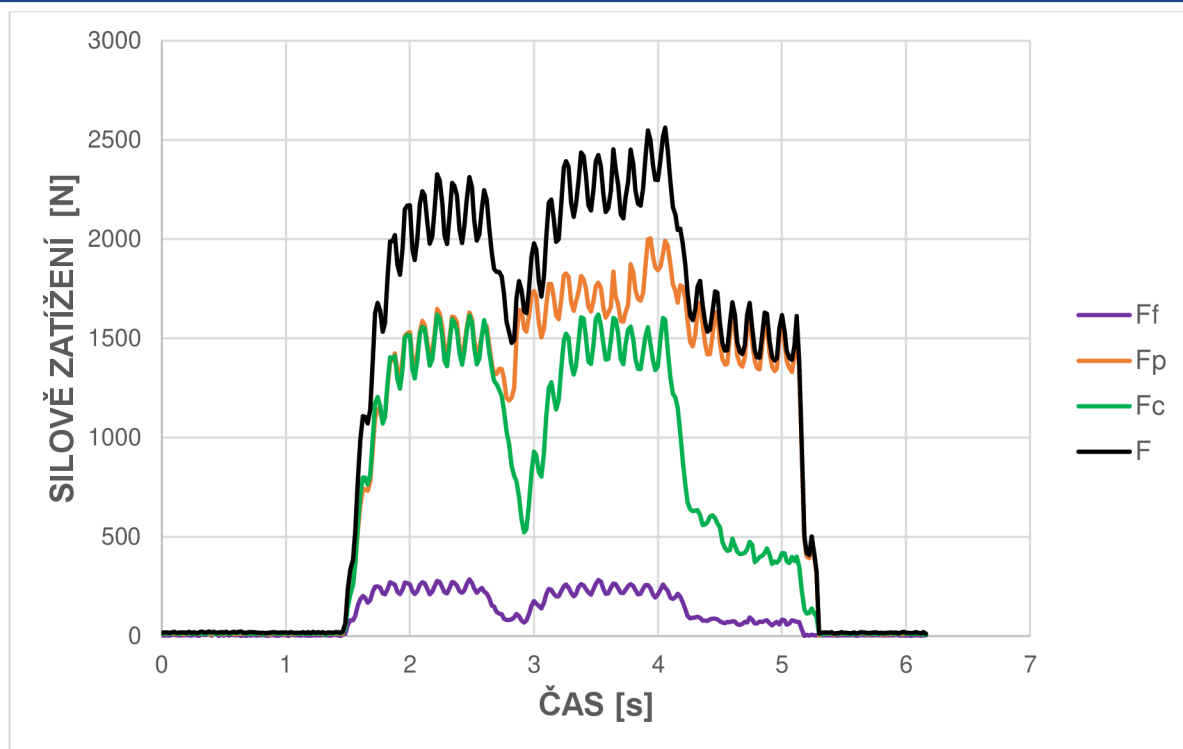
Obr. 3.40 Silové zatížení, VBD 7.
