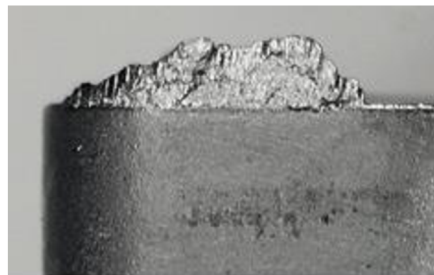
Obr. 2.9 Nárůstek na čele nástroje [1; 2].
