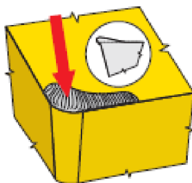
Obr. 2.9 Nárůstek na čele nástroje [1; 2].
