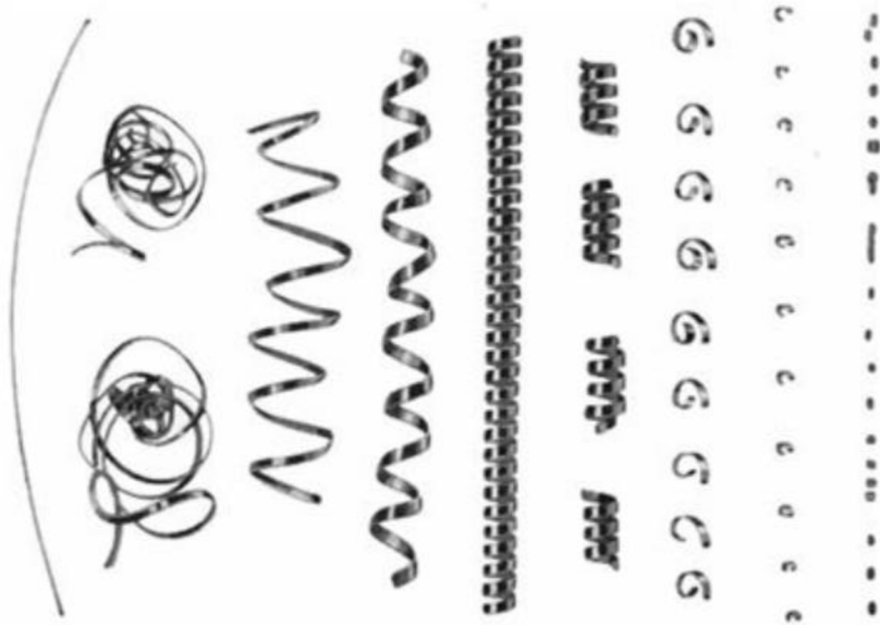
Obr. 2.3 Typy třísek [7].
