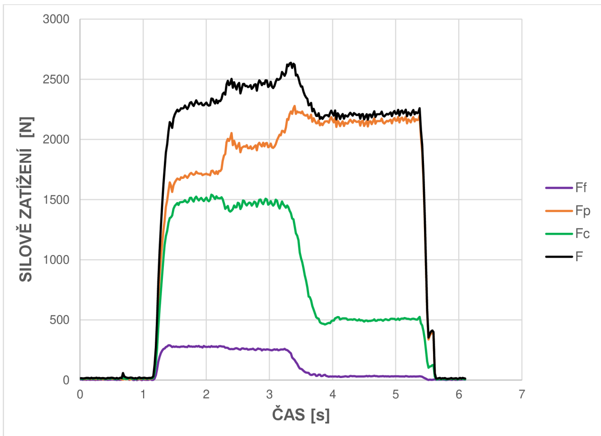
Obr. 3.35 Silové zatížení, VBD 2.
