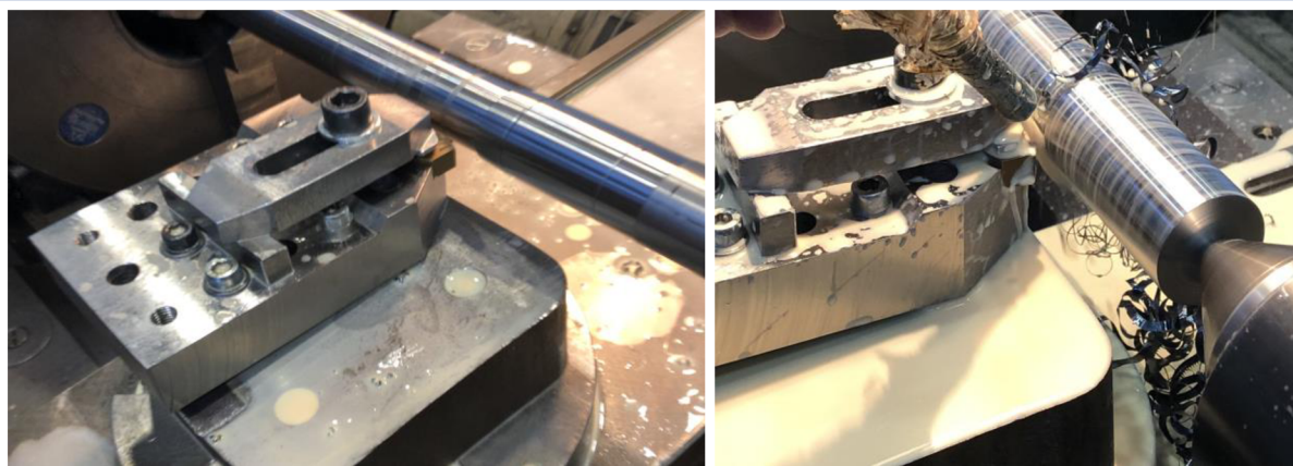
Obr. 3.22 Upnutí břitové destičky při stanovení řezných podmínek.
