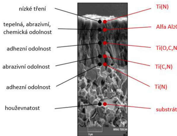
Obr. 2.17 Vícevrstvý povlak [21].
