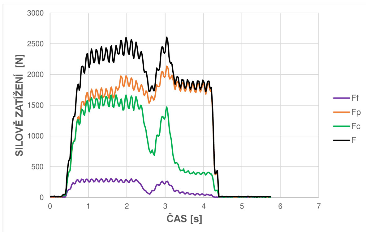
Obr. 3.41 Silové zatížení, VBD 8.
