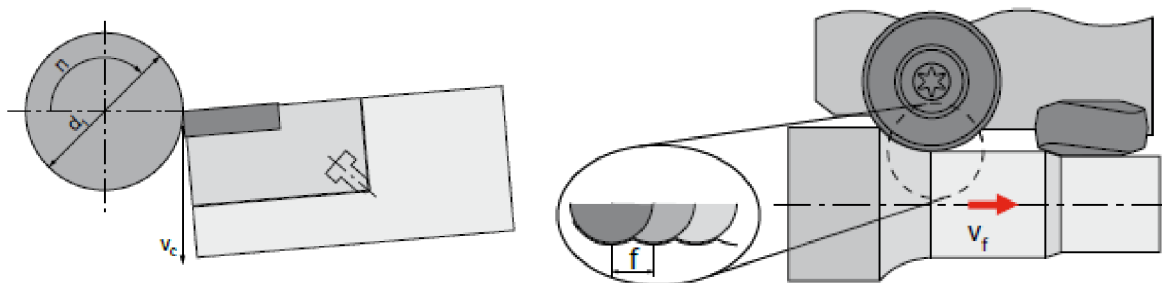
Obr. 1.14 Označení parametrů [1].
