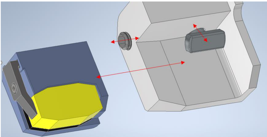
Obr. 4.3 Výměna kazety v držáku nástroje.
