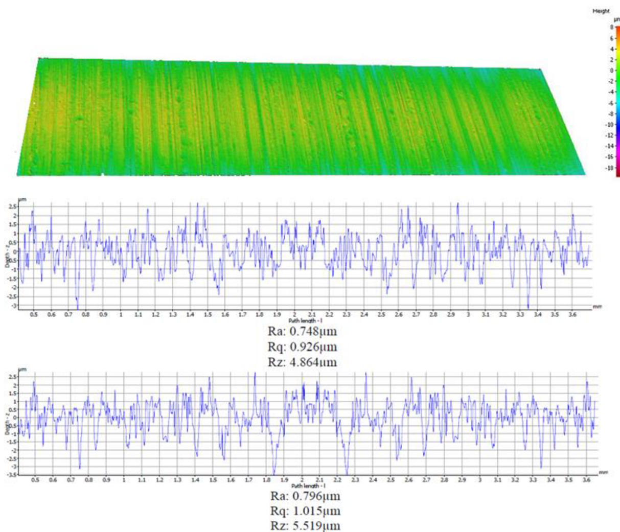
Obr. 3.20 Textura povrchu po kalibrační zkoušce pro VBD – A (horní), B (spodní).
