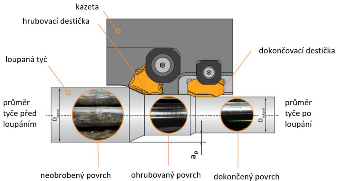
Obr. 1.10 Celková hloubka řezu [2].
