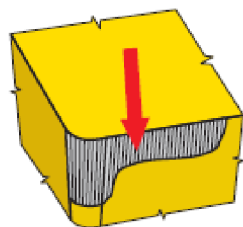
Obr. 2.8 Opotřebení hřbetu [1; 2].
