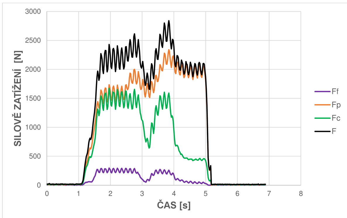
Obr. 3.39 Silové zatížení, VBD 6.
