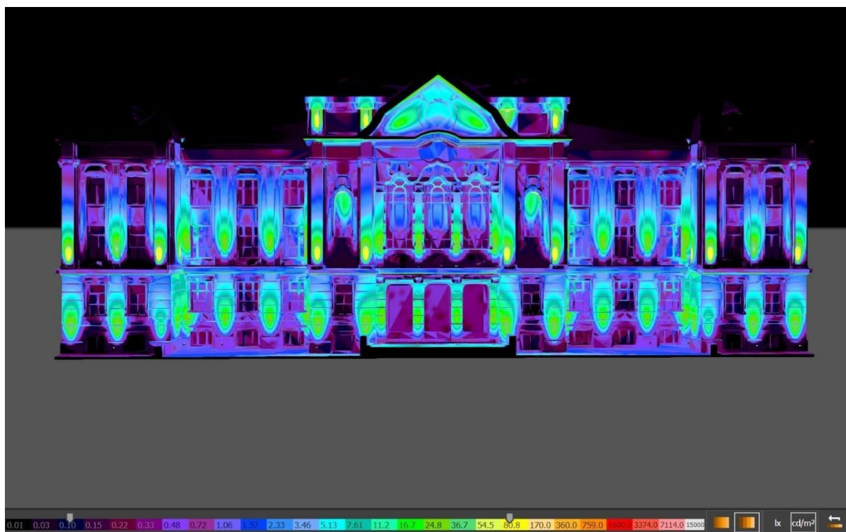
Obr. 14. Simulace jasu v programu DIALux evo
