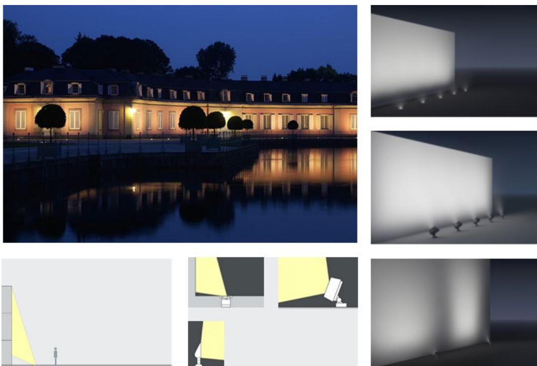
Obr. 3. Příklad wallwashing – plošné vertikální osvětlení z odstupu
