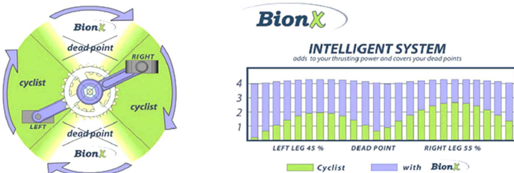
Obr. 6 Poměr pohonu motoru a cyklisty v systému BionX [26]
