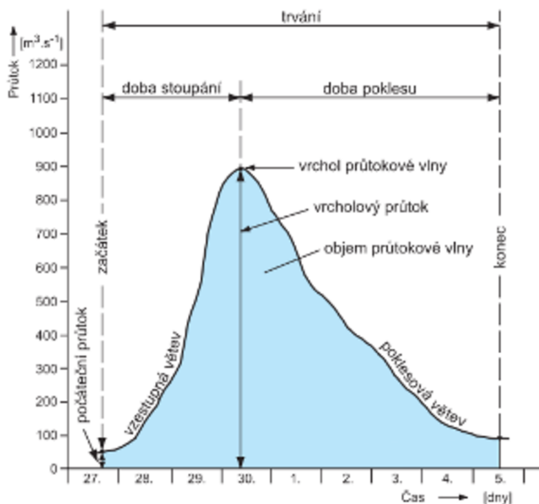
Obrázek 1: Hydrogram průtokové vlny a její prvky (upraveno podle ČSN, 1975, 1983) převzato od Brázdil, 2005.
