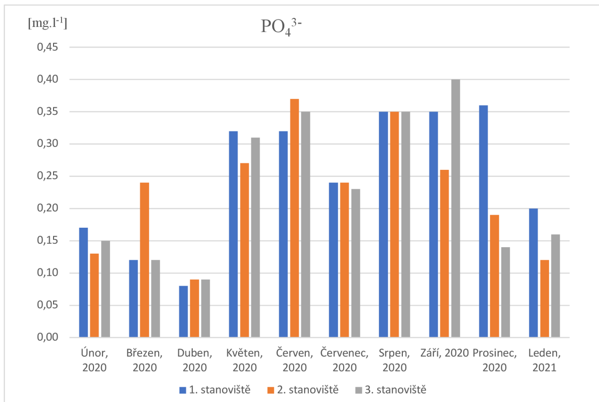
Obrázek 13: Koncentrace fosforečnanů
