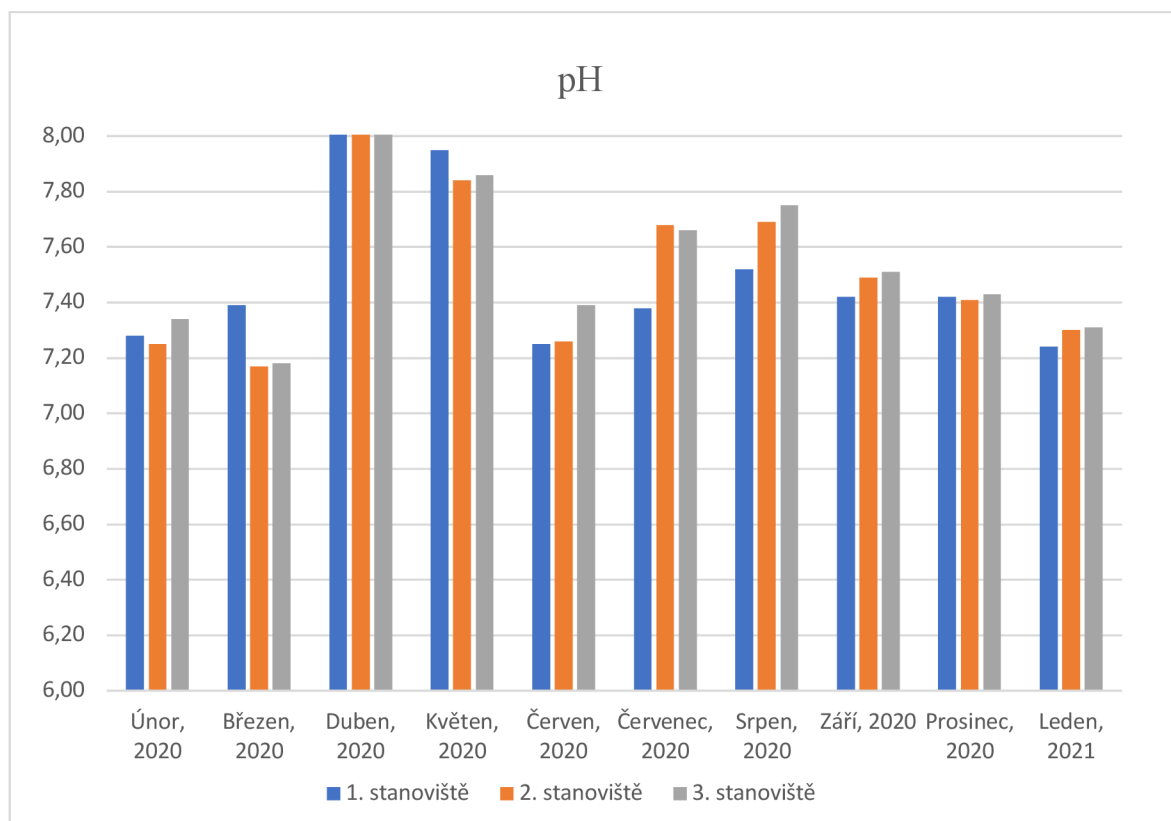
Obrázek 14: Hodnoty pH
