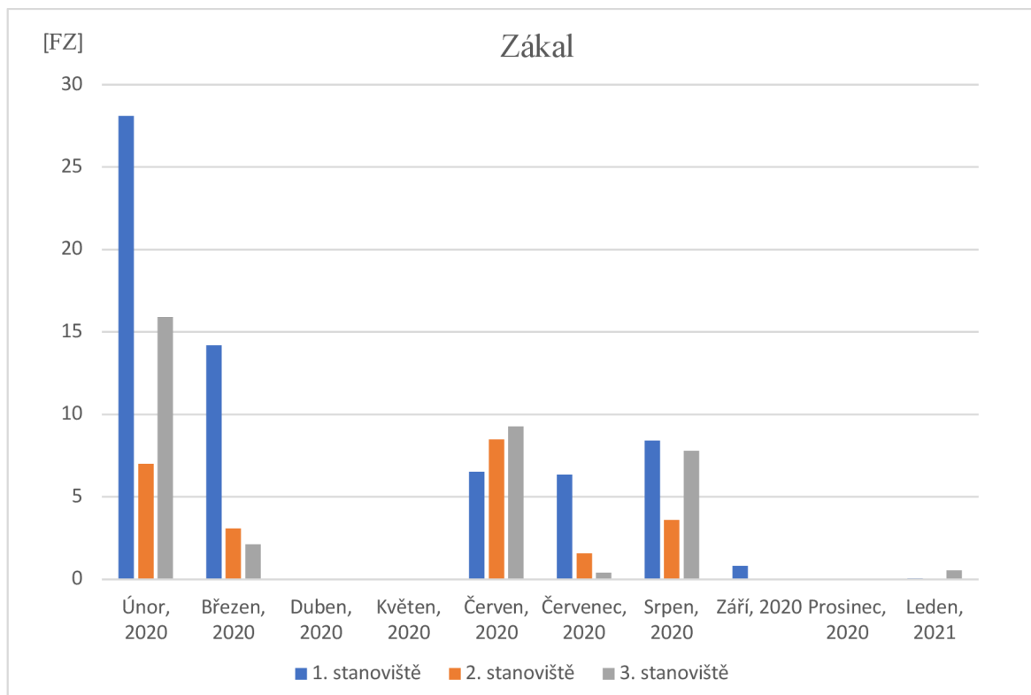
Obrázek 15: Hodnoty zákalu
