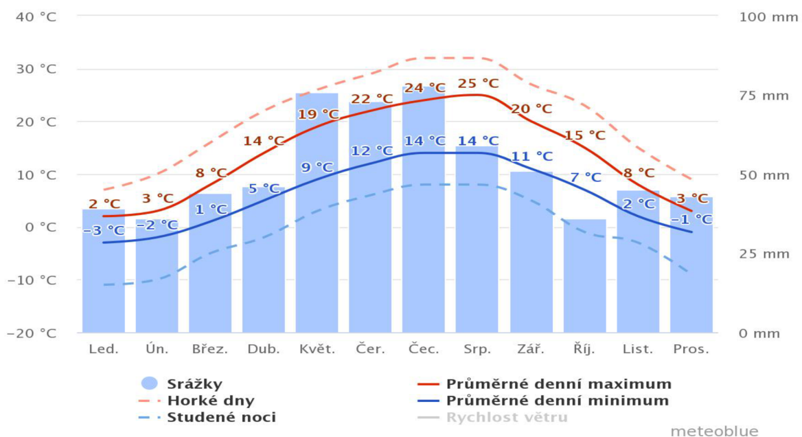
Obrázek 9: Klimatické poměry
