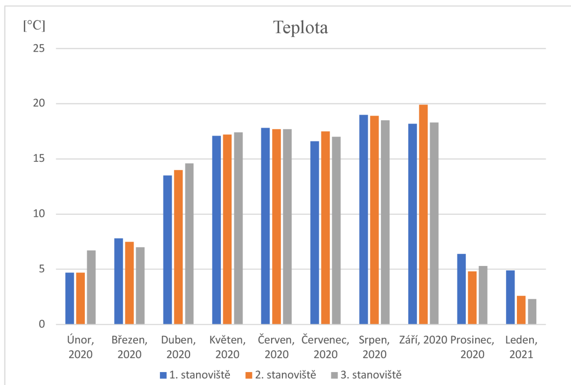
Obrázek 16: Teploty vody
