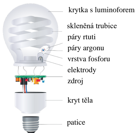
Obr. 2-14 Schéma zářivky, upraveno podle [30]
