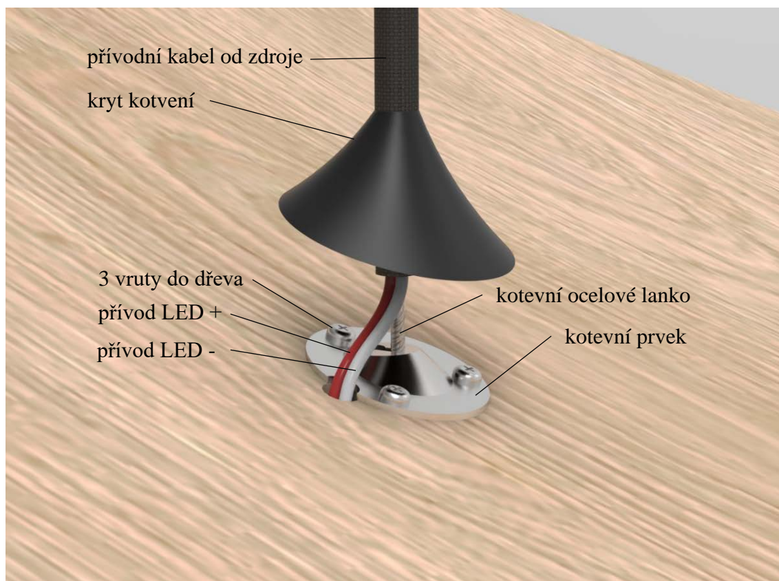
Obr. 6-11 Detail, kotvení nosné desky
