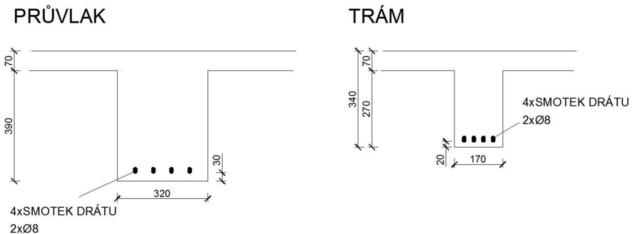
obr.8 ( rozměry a vyztužení prvků)
