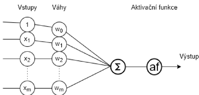
Obrázek 3.2: Schéma neuronu
