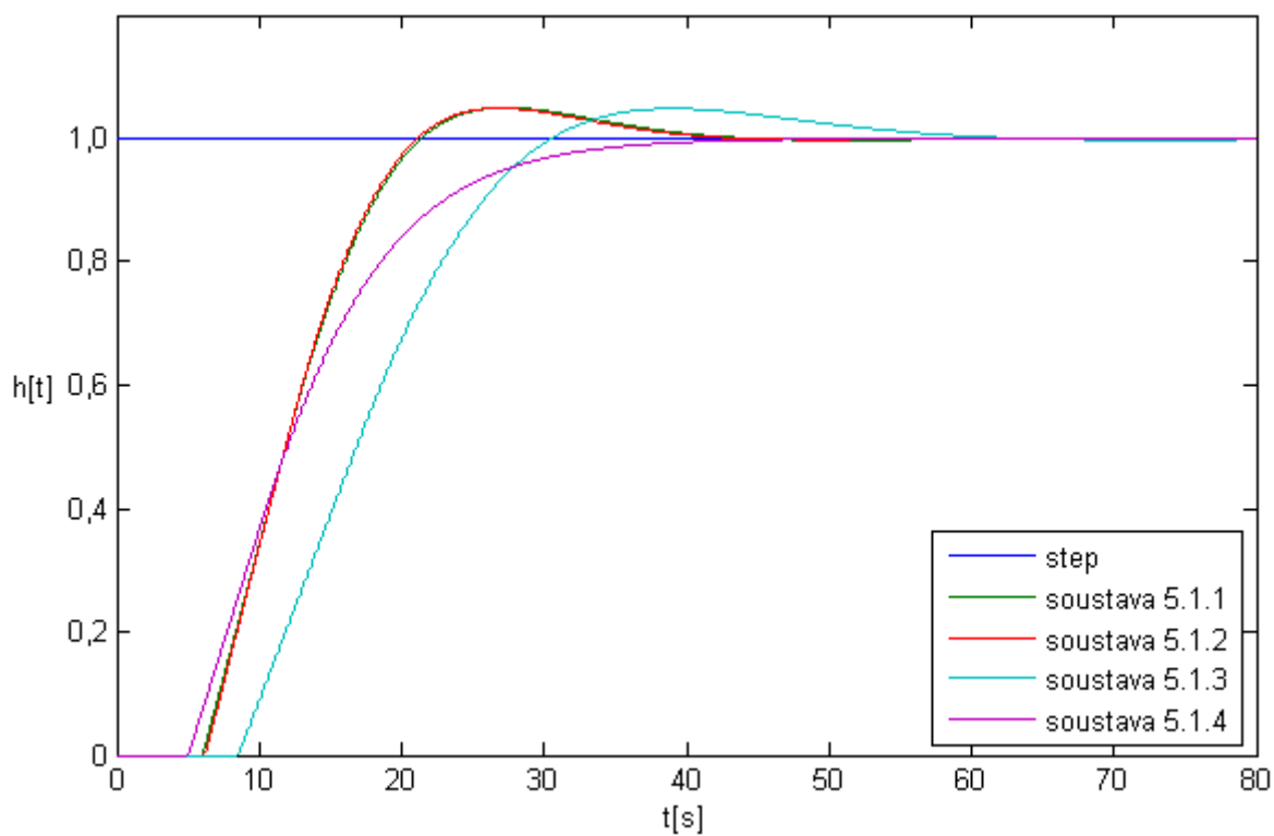
Graf 5.2 zobrazení průběhů regulace úprav soustavy 5.1
