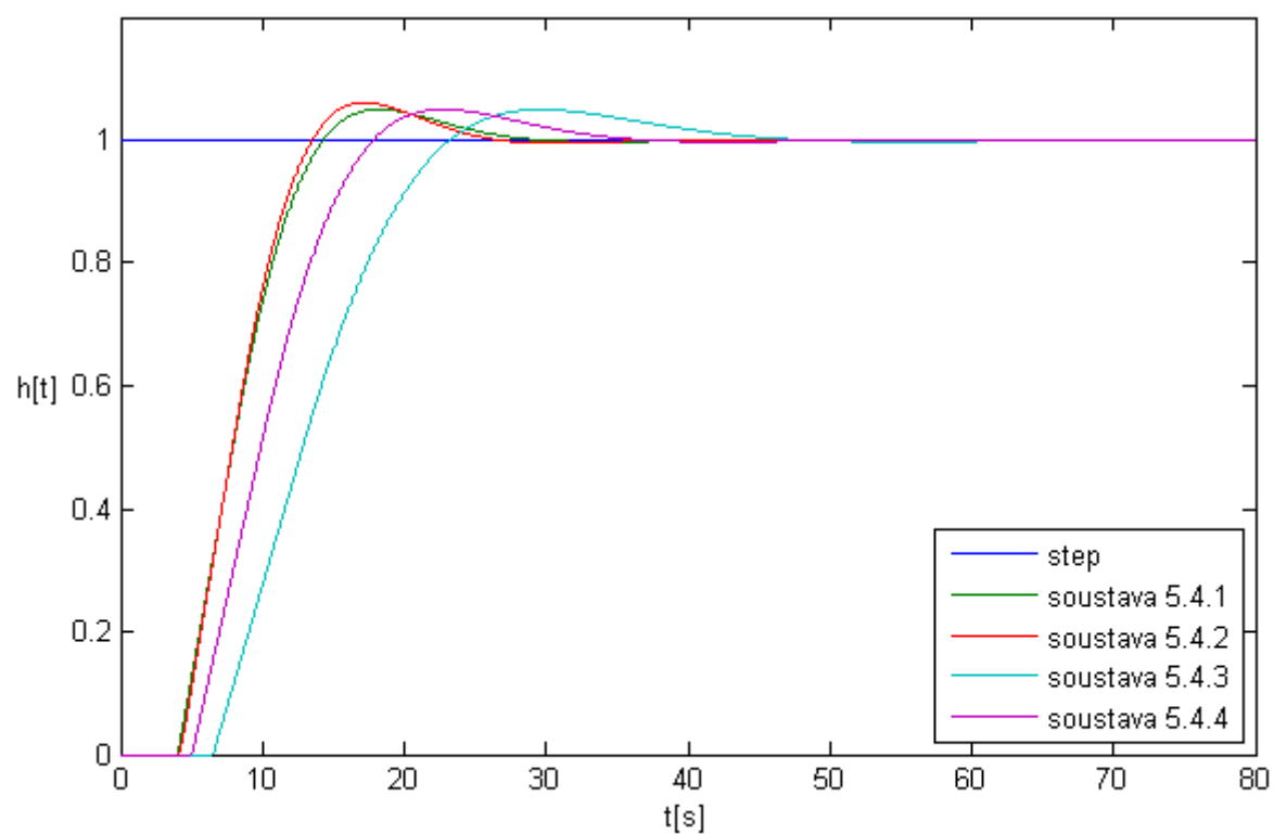
Graf 5.8 zobrazení průběhů regulace úprav soustavy 5.4
