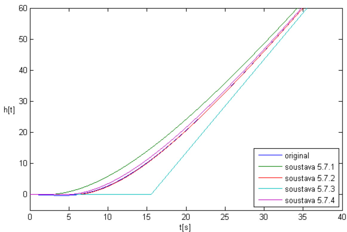
Graf 5.13 zobrazení přechodových charakteristik úprav soustavy 5.7
