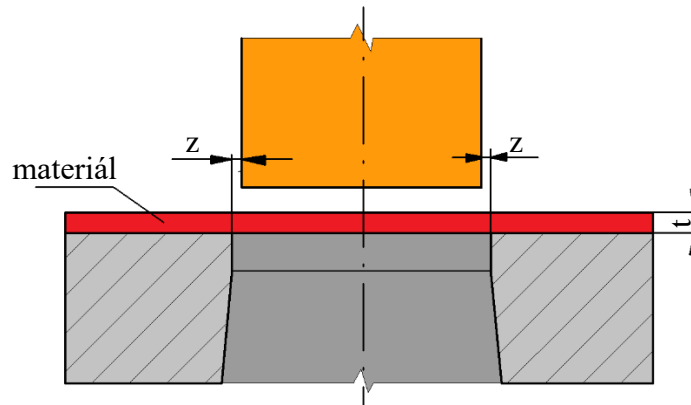
Obr. 18 Střižná mezera [26].
