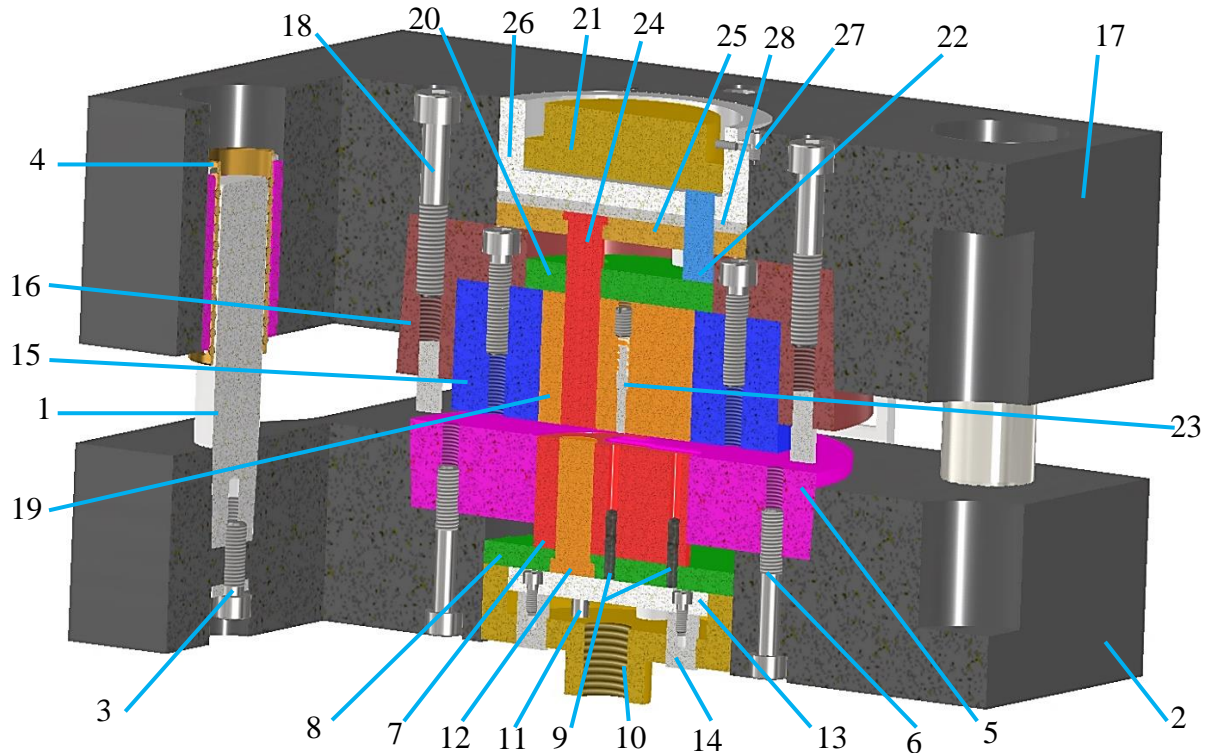
Obr. 38 Řez nástrojem.
