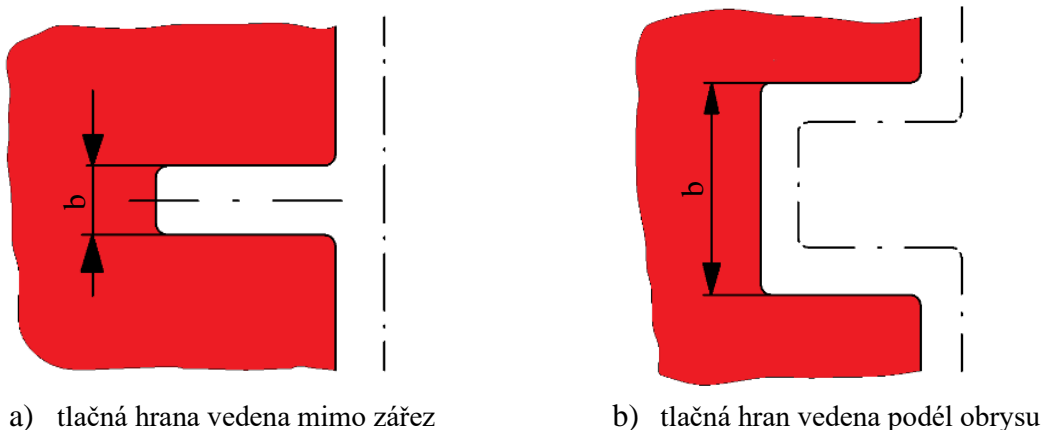
Obr. 15 Vedení tlačné hrany [20].
