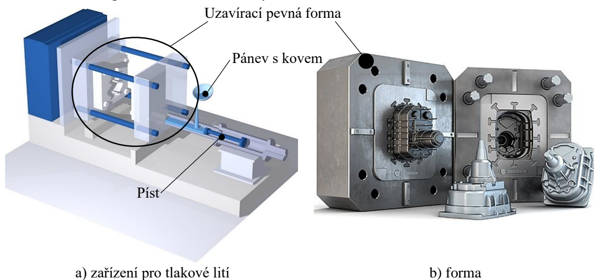
Obr. 4 Tlakové lití [23; 30].
