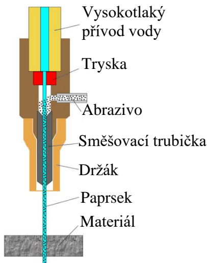
Obr. 5 Řezací hlava [9].
