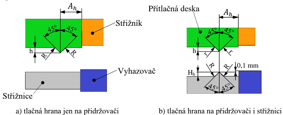
Obr. 14 Tvar a vzdálenost tlačné hrany od kraje [16].
