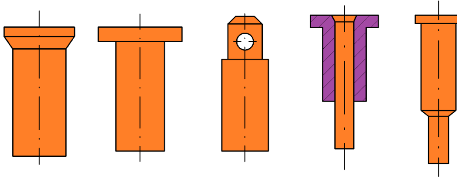
Obr. 25 Upínání střížníků [15].
