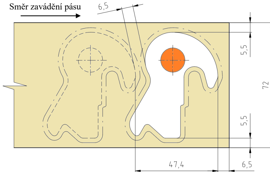
Obr. 31 Varianta A.
