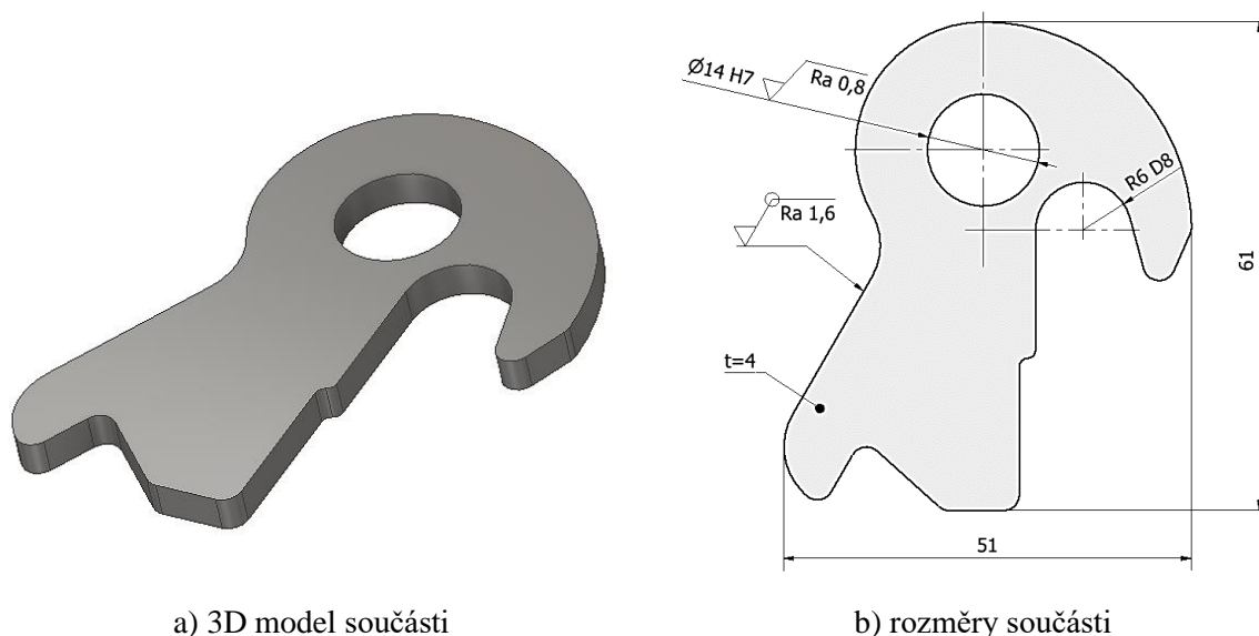
Obr. 3 Vyráběná součást.
