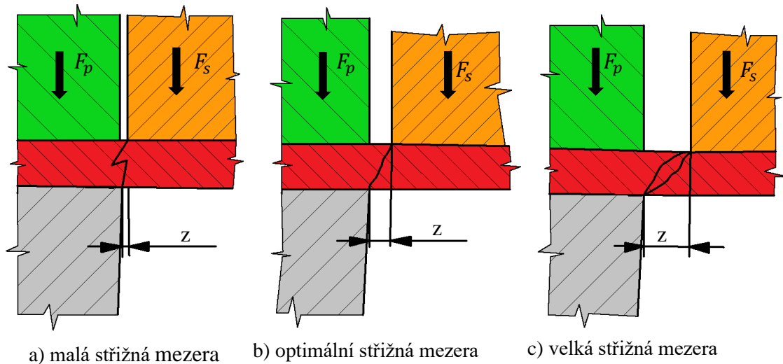
Obr. 19 šíření trhliny [25].
