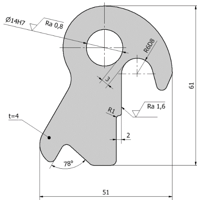
Obr. 29 Segment zámku.
