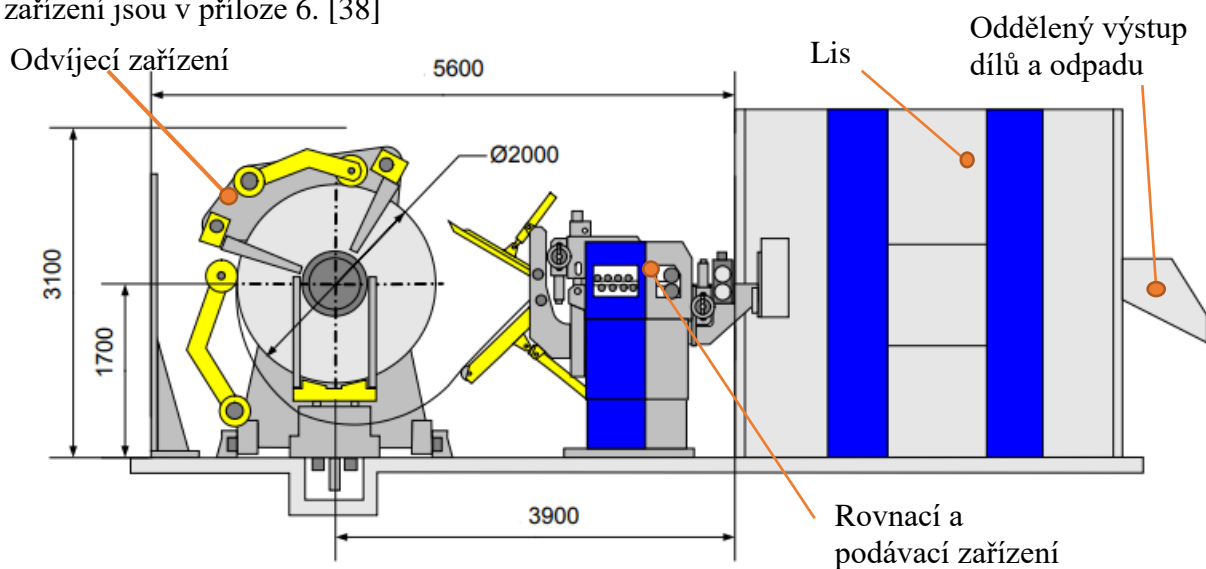
Obr. 40 Stříhací linka [38].
