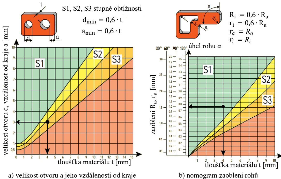
Obr. 30 Použité nomogramy [16].
