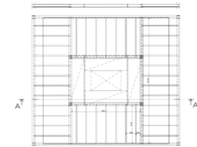
STROP_03 Kavárna
