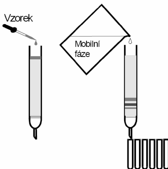
Obr. č. 5: Schéma základního experimentálního uspořádání LSC [46]
