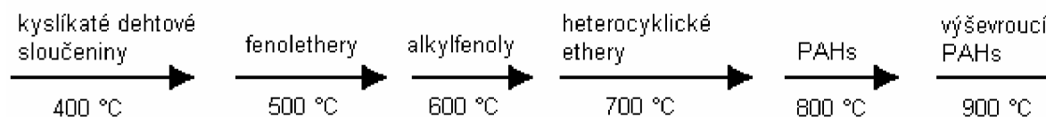
Obr. č. 1: Schématické znázornění tvorby dehtu při spalování biomasy [7]
