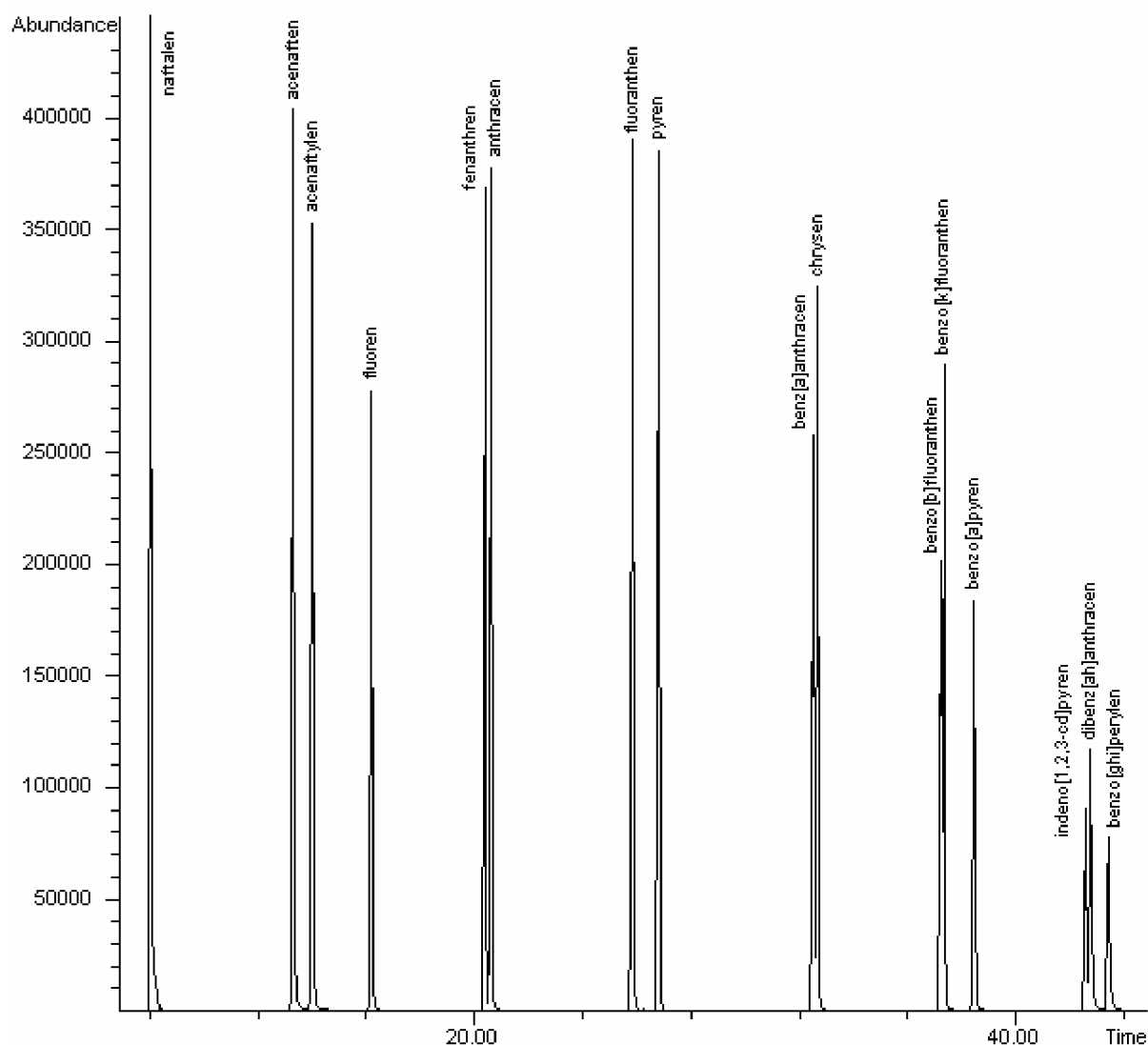
Obr. č. 11: Chromatogram standardu PAH – Mix 9 o koncentraci 20 \mu\text{g/ml}
