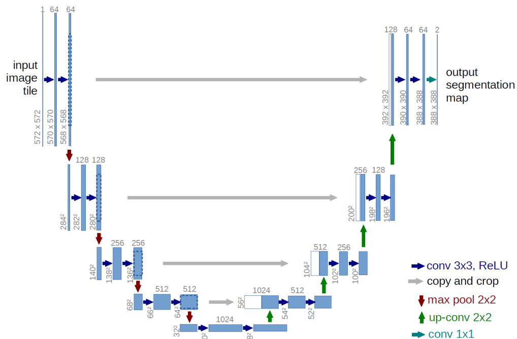
Obr. 1.2: Původní architektura U-Net [12]
