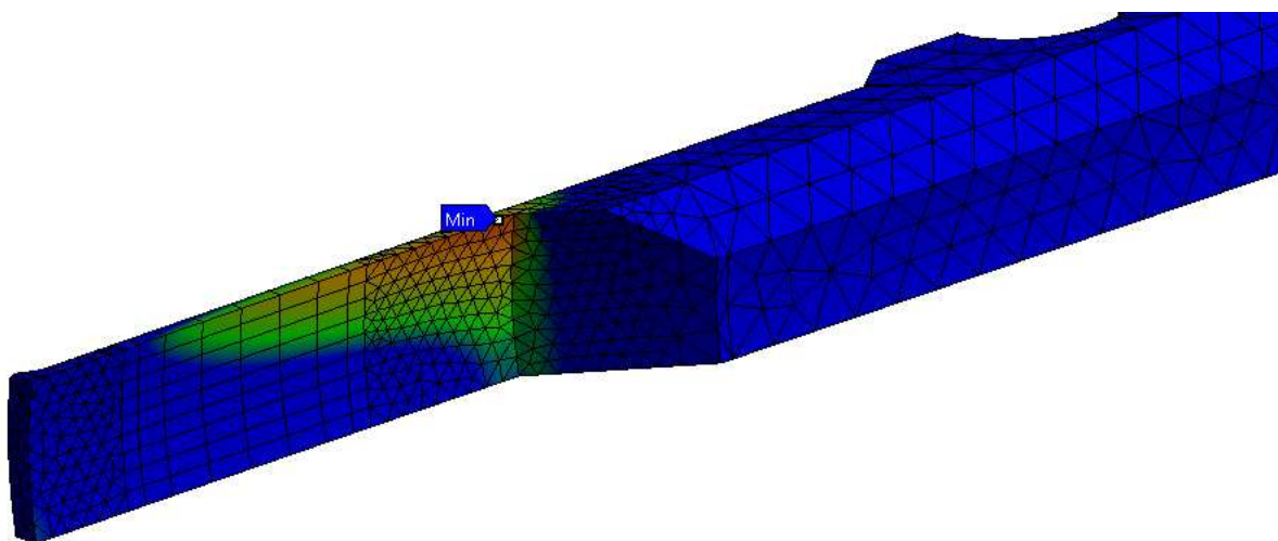
Obr. 69 Bezpečnost pro 1 milion zátěžných cyklů
