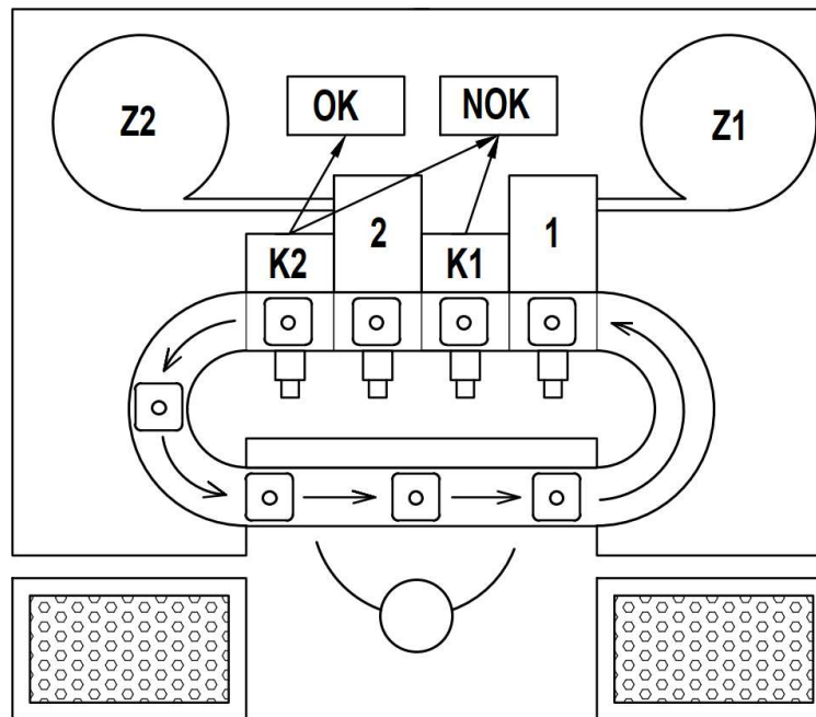
Obr. 73 Schéma Varianty 1
