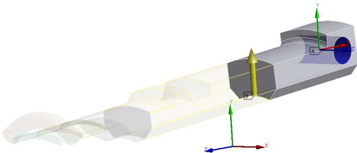
Obr. 63 Okrajové podmínky
