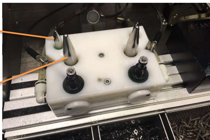
Obr. 16 Navlékací trny
