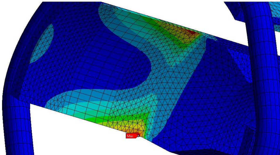
Obr. 64 Maximální napětí
