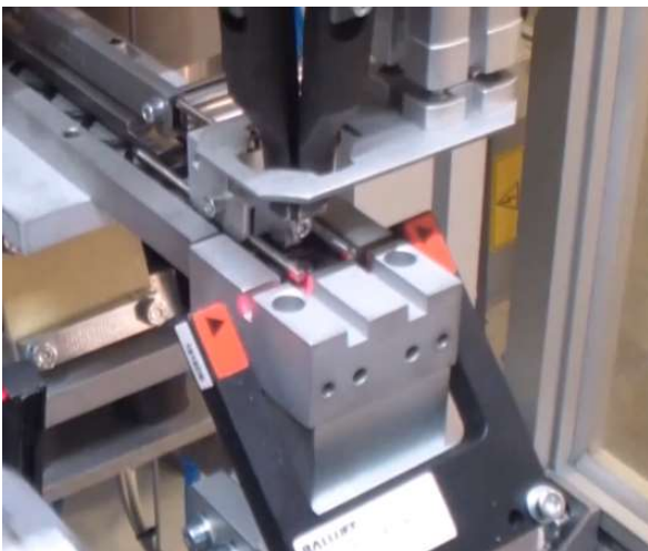
Obr. 43 1. Hlava s chapadly čekající na příjezd výtahu s o-kroužkem [15]
