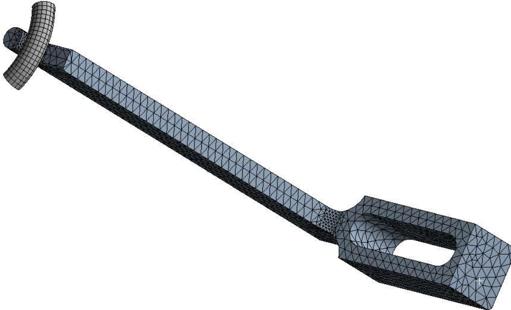
Obr. 49 Síťování chapadla
