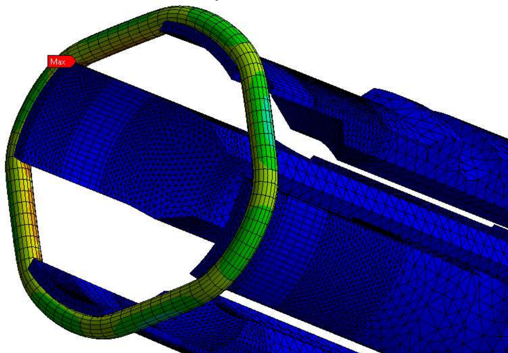
Obr. 65 Napjatost
