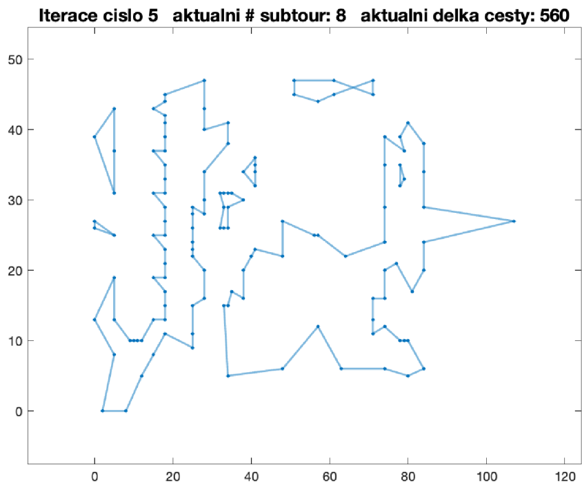
Obrázek 7: V. iterace - 131 uzlů VLSI
