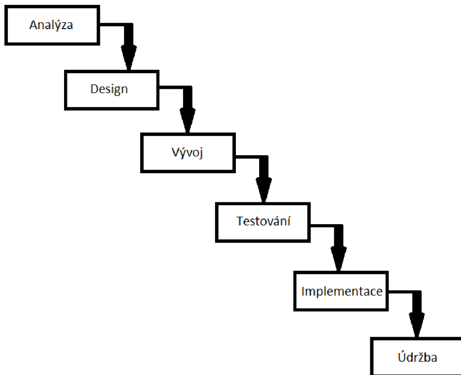
Obrázek 1: Vodopádový model
