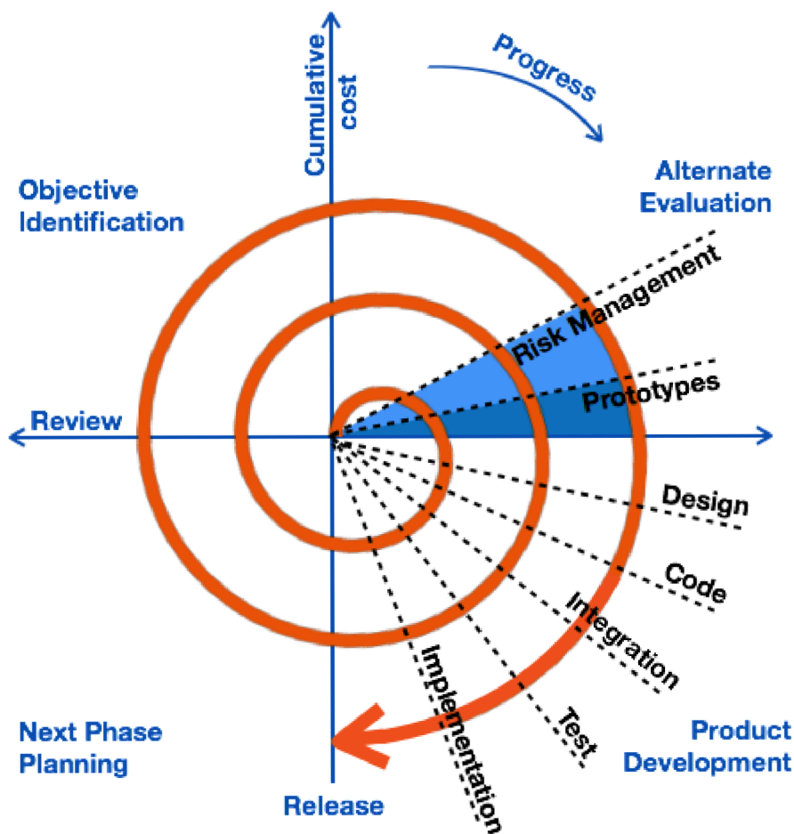
Obrázek 3: Spirálový model
