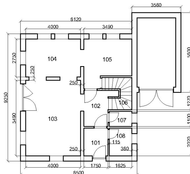
Obrázek 2: Přízemí
