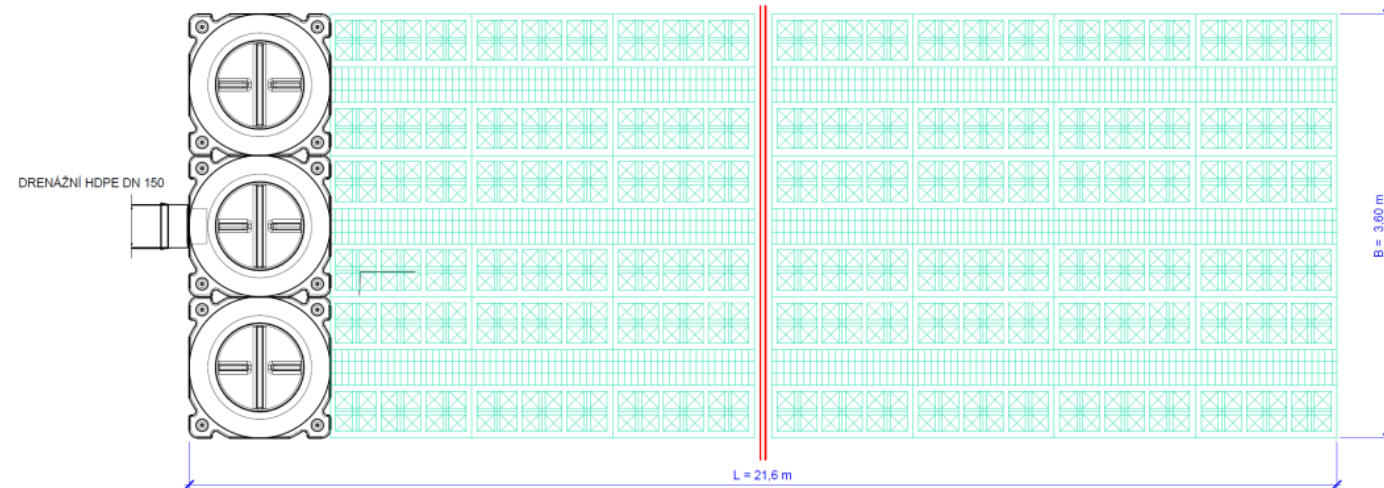
PŮDORYS
