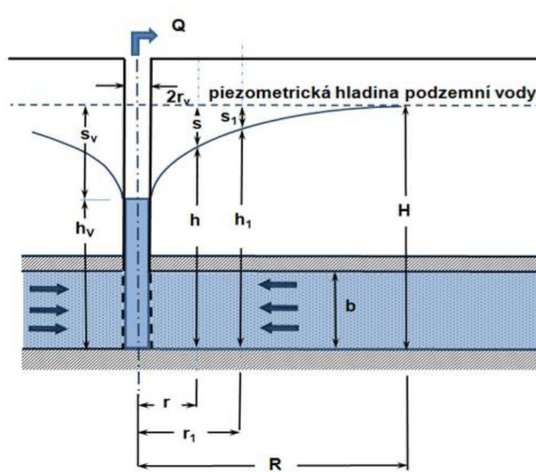
Obrázek 2: Ideální vrt (Pech, 2015)
