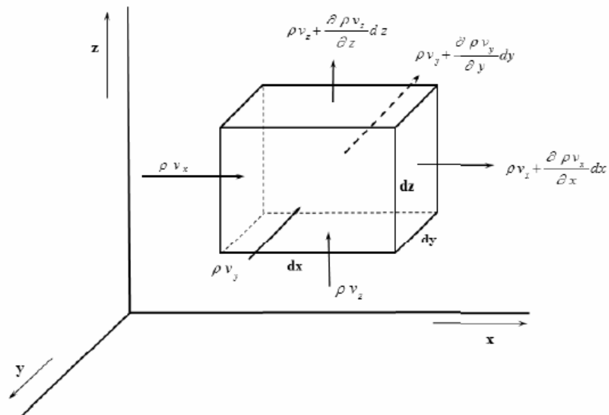
Obrázek 5: Elementární rovnoběžnostěn (Pech, 2010)
