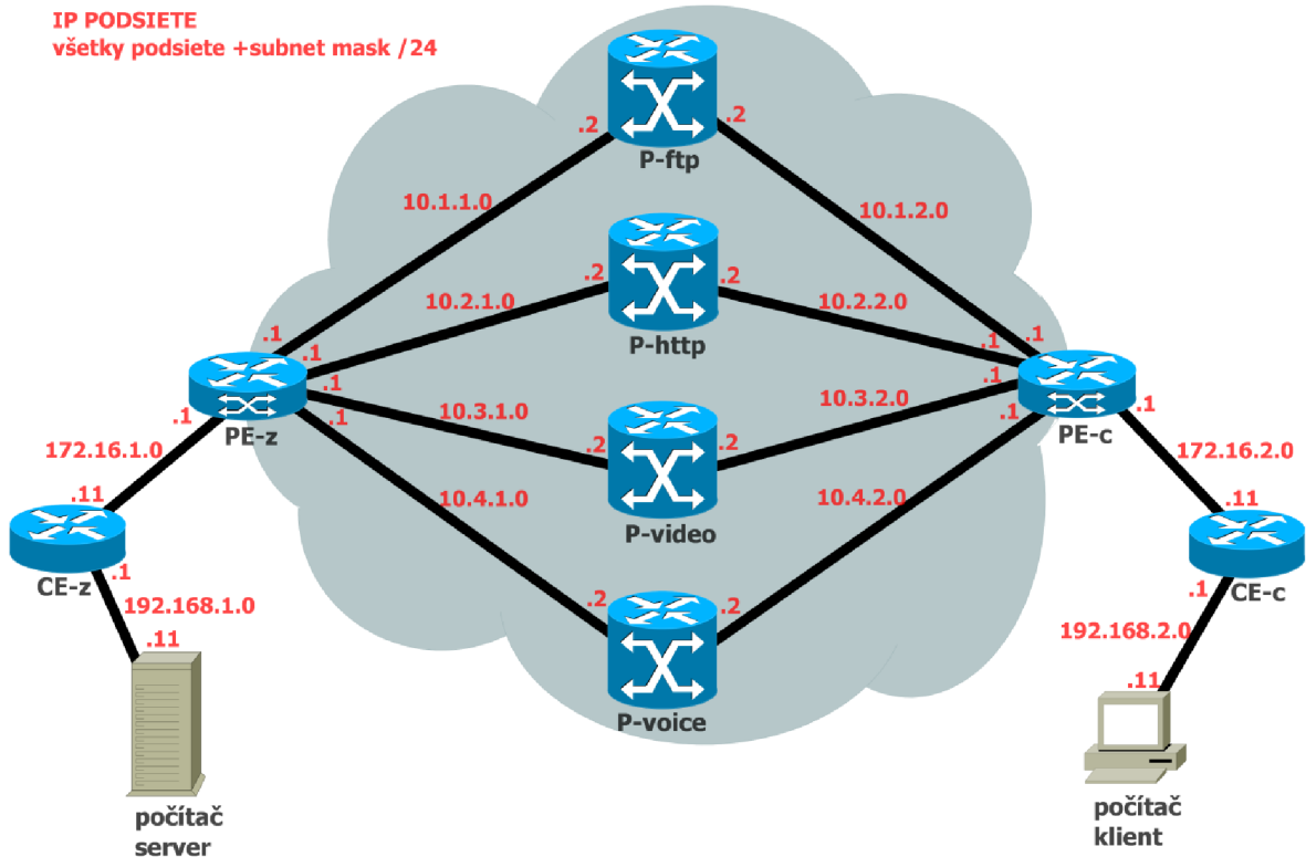
Obr. 8: Plán IP adresovania
