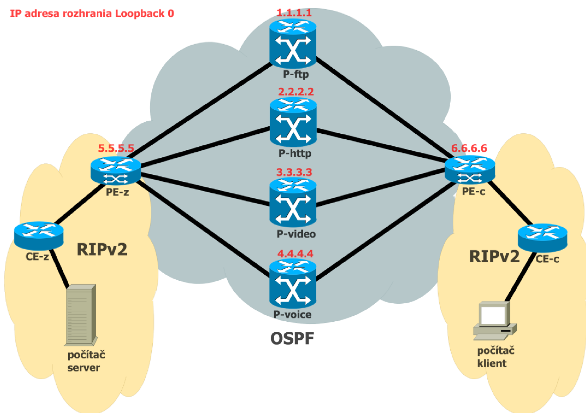
Obr. 9: Smerovacie domény
