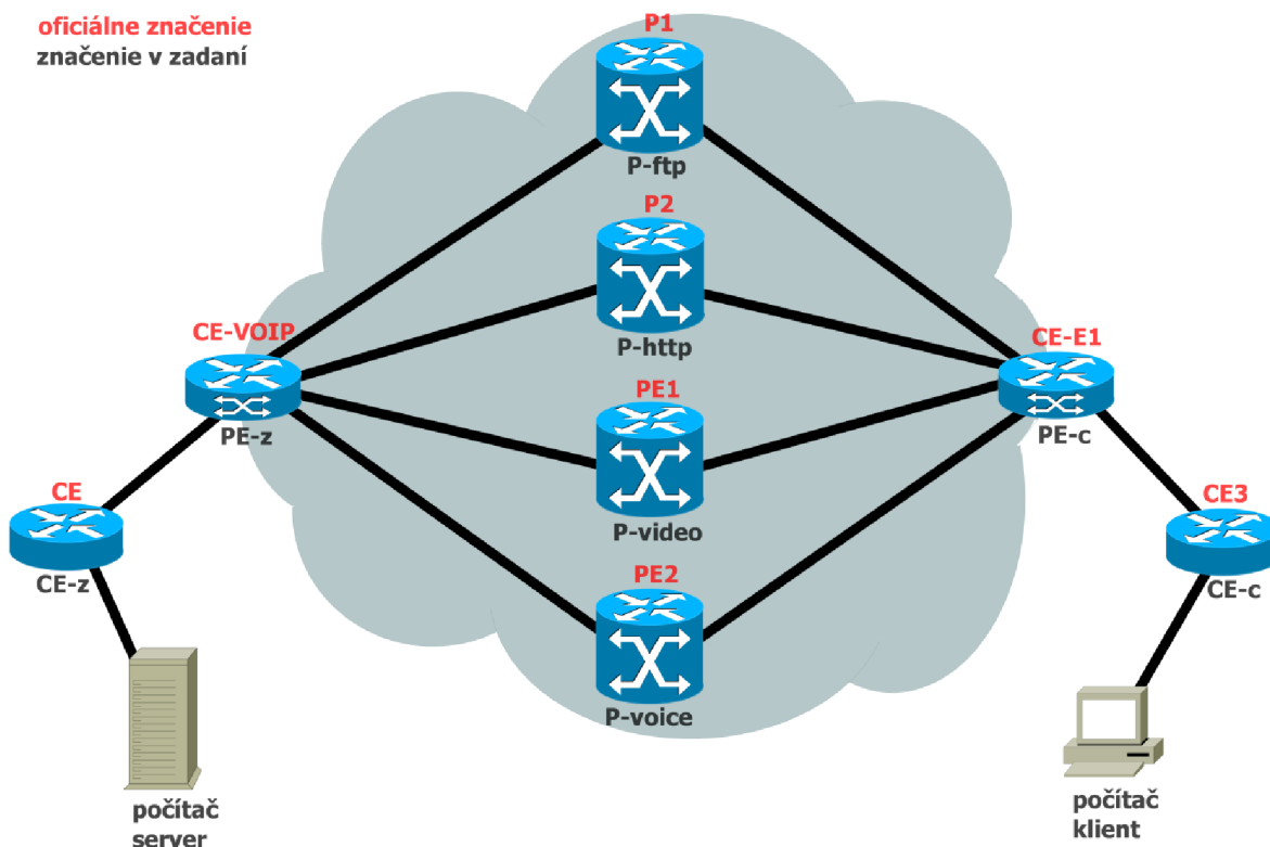
Obr. 6: Použité smerovače
