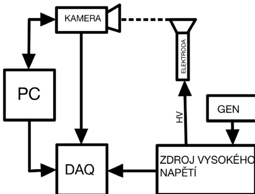
Obrázek 22: Schéma experimentálního uspořádání sestávající se z elektrody s šroubovu rotační pumpou obsahující polymerní roztok v zásobníku, vysokonapěťového zesilovače (TREK) s generátorem signálu (GEN-Owon AG 1022), vysokorychlostní kamery (i-SPEED 720), systému pro sběr dat (8-kanálový DAQ převodník NI USB-6216) a počítačem (PC) [6].
