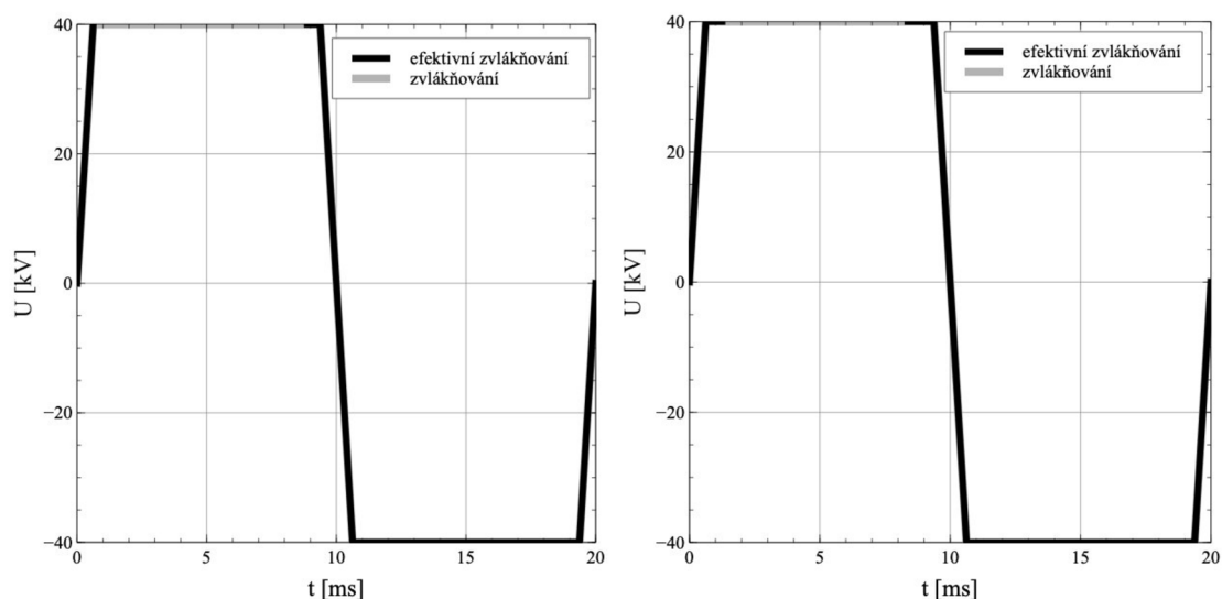
Obrázek 33: Zvlákňovací procesy AC elektrického zvlákňování řízené obdélníkovým vysokonapětovým signálem pro roztok PVB 12 % statický (vlevo) a dynamický (vpravo). Napětové signály jsou znázorněny šedými kružnicemi, zvlákňovací oblasti jsou zobrazeny jako plná šedá čára a efektivní oblasti elektrického zvlákňování jsou zvýrazněny plnými černými čarami.
