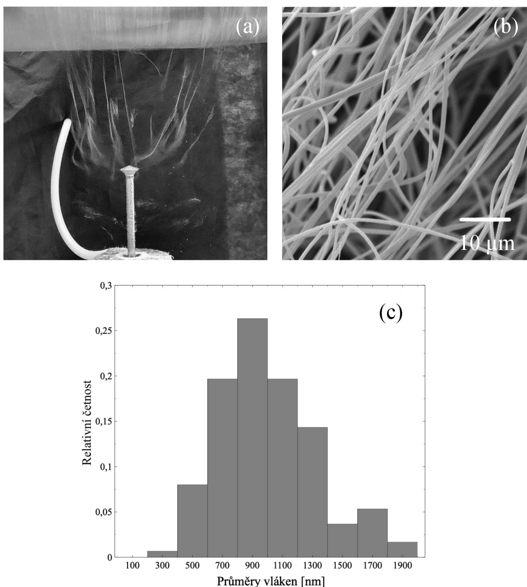
Obrázek 39: Nanovláknenná vlečka (a), nanovláknenná vrstva (b), histogram relativních četností průměrů PVB 12 % VN obdélníkového signálu (c)
