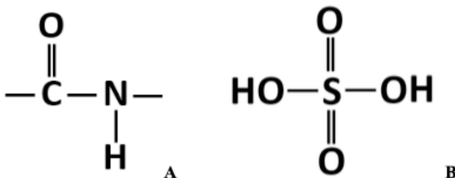
Obrázek 11: Amidová vazba obsažená v PA 6 (A). Příklad kyseliny (B) sloužící jako aditivum, konkrétně \text{H}_2\text{SO}_4 disociující do prvního i druhého stupně ve vodném prostředí [7].
