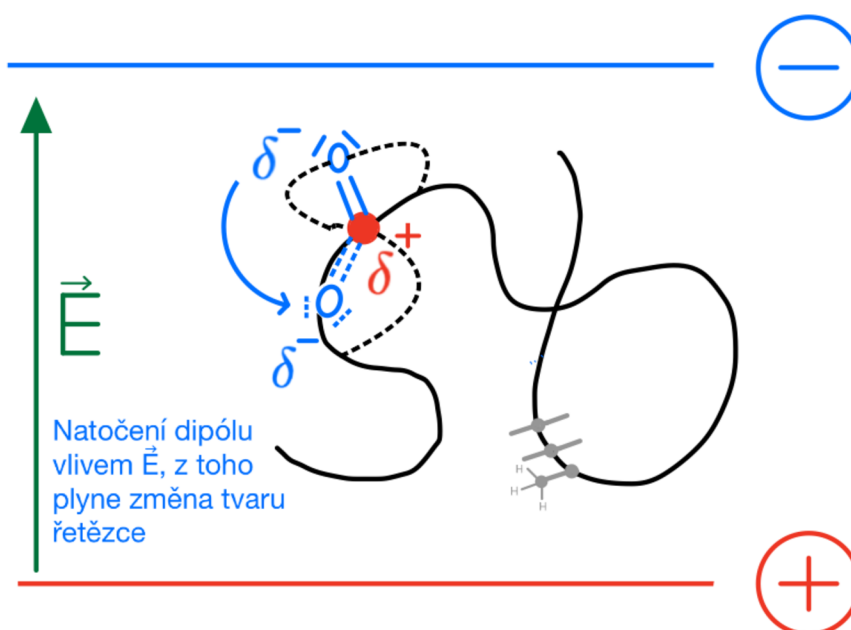
Obrázek 10: Makromolekula uvnitř elektrického pole (vlastní zdroj)
