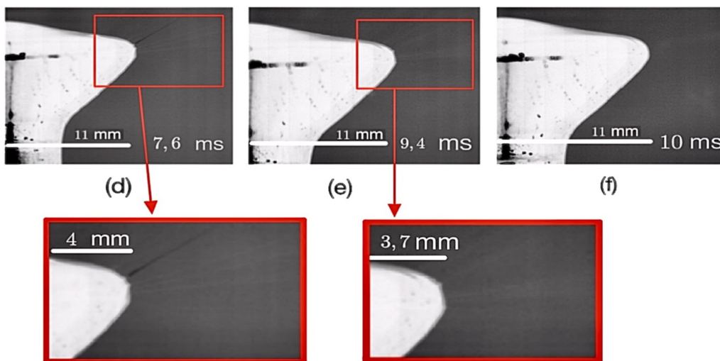
Obrázek 26: Sekvence snímků zobrazuje elektrické zvlákňování PVB 10 % s přeplavováním, kdy byl použit vysokonapěťový sinusový signál. Pouze zvlákňování (d), zhroucení trysek (e), oblast nezvlákňování (f) (vlastní zdroj).
