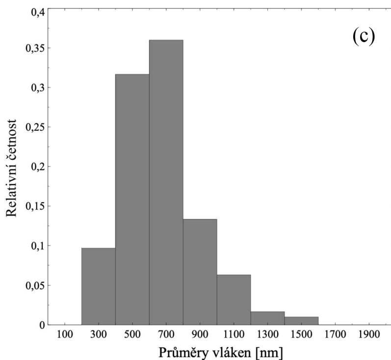
Obrázek 35: Nanovláknenná vlečka (a), nanovláknenná vrstva (b), histogram relativní četnosti průměrů PVB 11 % VN sinus (c)
