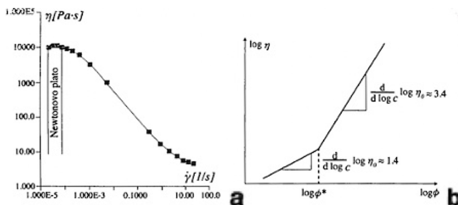
Obrázek 15: Newtonovo plato dynamické viskozity u při nízkých hodnotách smykového rychlosti \dot{\gamma} (a).
