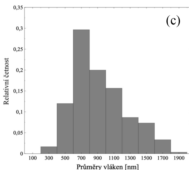
Obrázek 37: Nanovlákná vložka (a), nanovlákná vrstva (b), histogram relativních četností průměrů vláken PVB 10 % VN obdélník (c)
