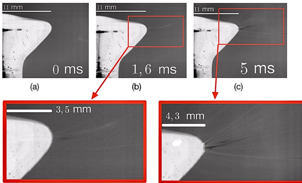
Obrázek 25: Sekvence snímků zobrazuje elektrické zvlákňování PVB 10 % s přeplavováním, kdy byl použit vysokonapěťový sinusový signál. Elektroda bez hydrodynamické nestability (a), generování prvních polymerních trysek (b), efektivní oblast zvlákňování (c) (vlastní zdroj).
