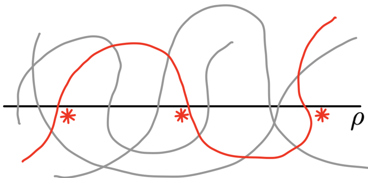
Obrázek 12: Model řetězce polymeru obtáčející rovinu \rho (přechody roviny jsou značené *) [33]
