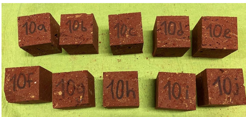
Obrázek 44, Zkušební vzorky cihly č. 10.
