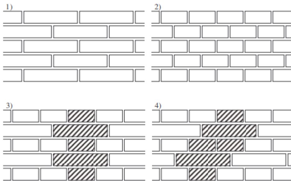
Obrázek 1, Typy používaných vazeb 1) běhounová, 2) vazáková, 3) polokřížová, 4) křížová [2].
