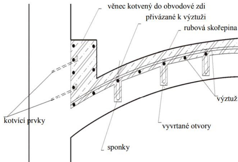
Obrázek 15, Možné řešení rubové skořepiny [6].
