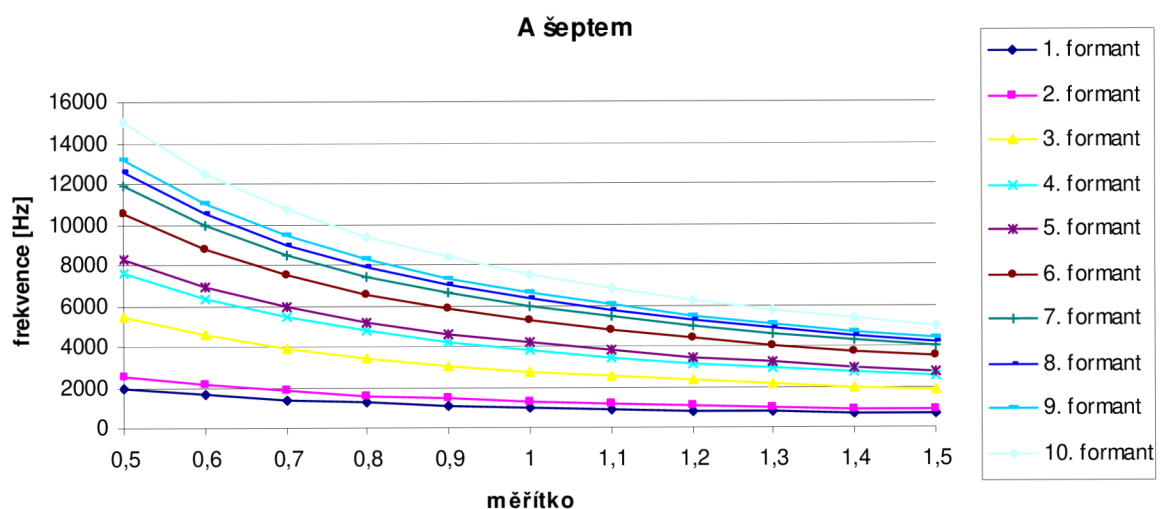
Obr. 9.8 Závislost frekvencí na velikosti vokálního traktu u samohlásky A šeptem
