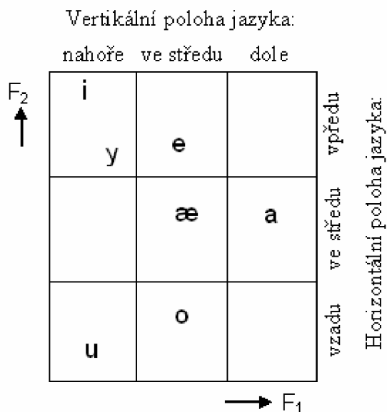
Obr. 6.1 Poloha prvních dvou formantů podle polohy jazyka
