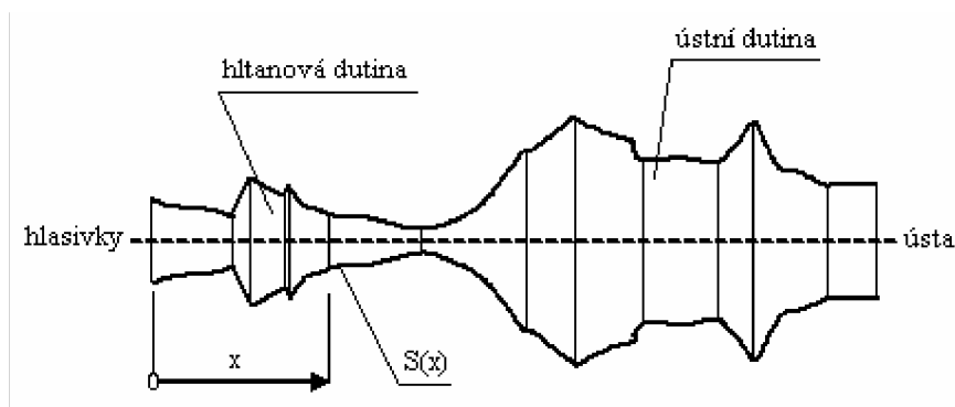
Obr. 5.2 Rotační model vokálního traktu pro samohlásku A
