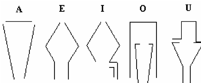
Obr. 3.1 Kratzensteinův rezonátor [8]
