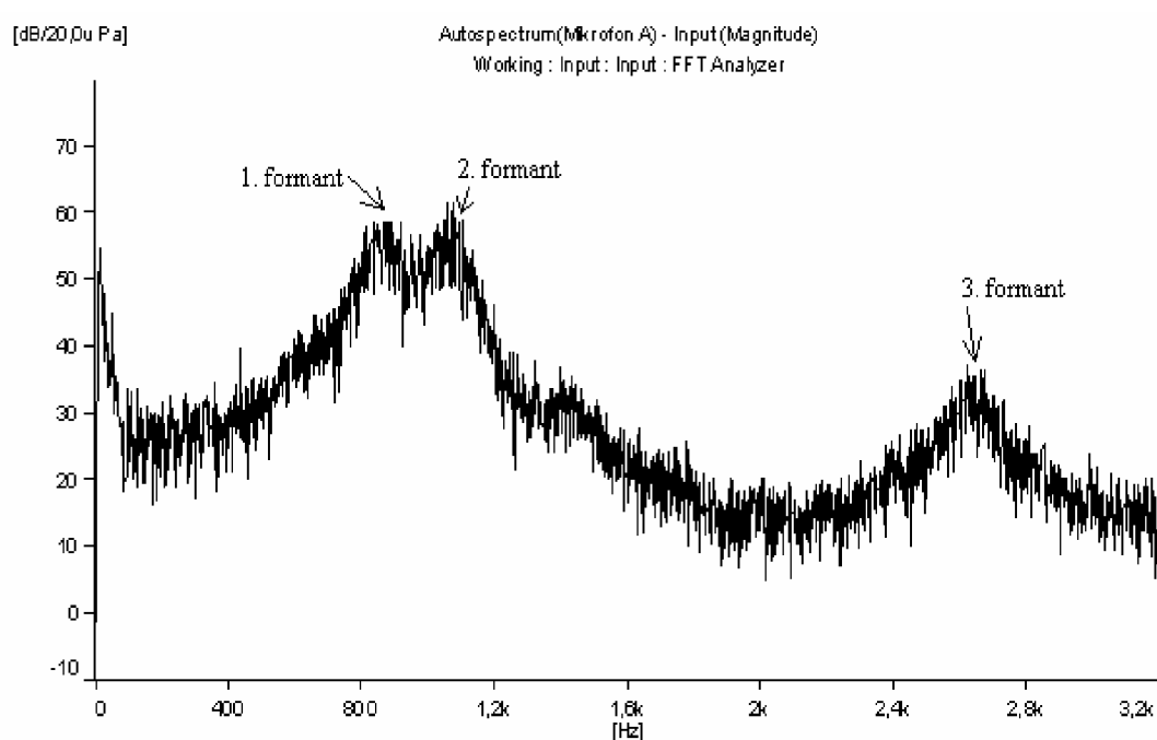
Obr. 11.5 Autospektrum samohlásky A vyslovené šeptem
