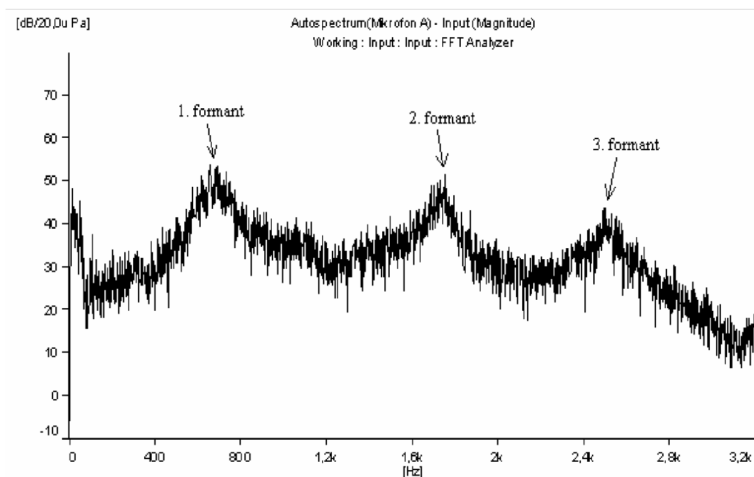
Obr. 11.6 Autospektrum samohlásky E vyslovené šeptem
