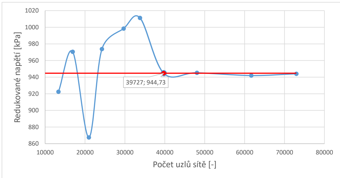
Obr. 34 Konvergence sítě
