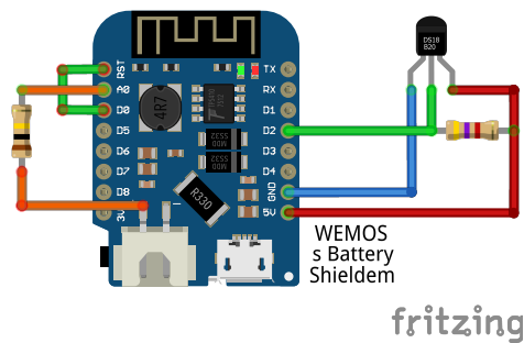
Obrázek 4.12: Schéma zapojení komponenty pro měření teploty. Jedná se o pospojování jednotlivých součástí, tak jak jsou zapojeny ve finální podobě zařízení.
