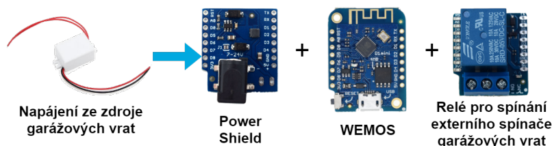
Obrázek 3.7: Blokové schéma ovládání garážových vrat. Deska WEMOS napájena ze zdroje garážových vrat a relé pro spínání kontaktu externího spínače garážových vrat.
